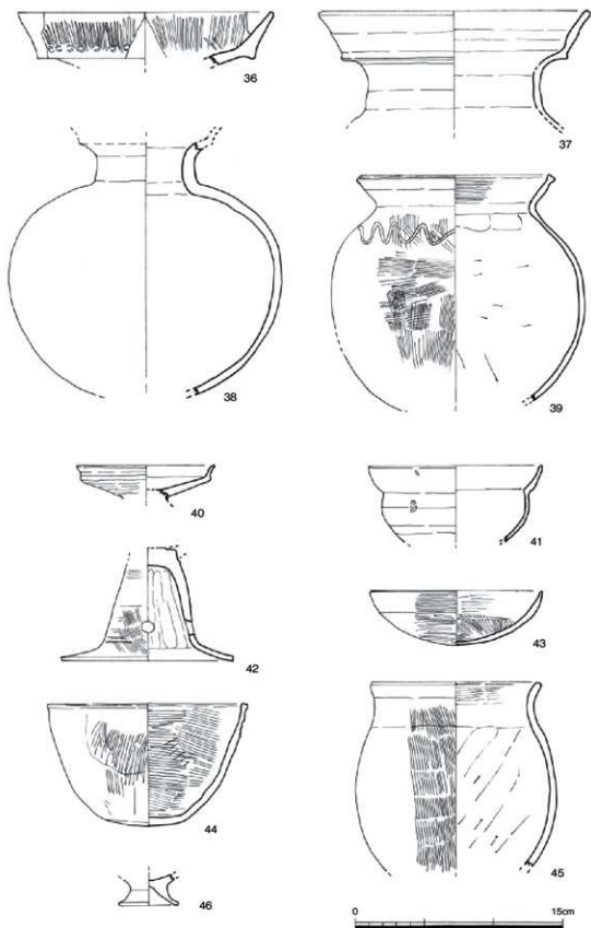
图13 SC99出土遺物実測図 (S = 1 / 3)
