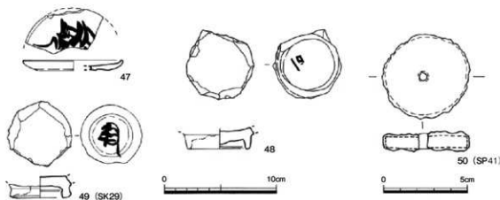
図14 その他の出土遺物実測図 (S = 1/3、1/2)
