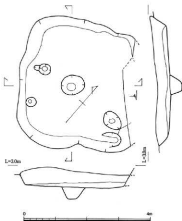
図12 SC99実測図 (S = 1/60)
