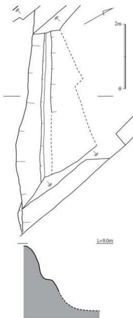
図 17 SX13 (S=1/60)
