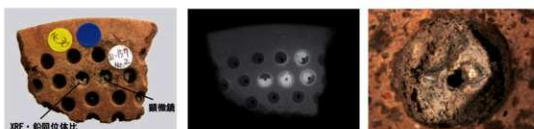
No. 18 (左) 資料写真 (中) CR画像 (右) 型穴内ガラス顕微鏡写真
