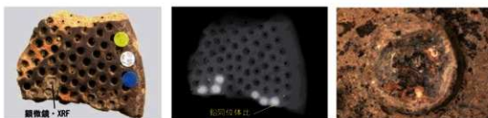
No. 16 (左) 資料写真 (中) CR画像 (右) 型穴内ガラス顕微鏡写真
