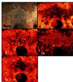
蛍光X線元素マッピング (No. 9)
