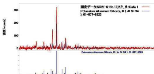
棒状土製品付着白色物質のX線回折スペクトル (No. 1)
