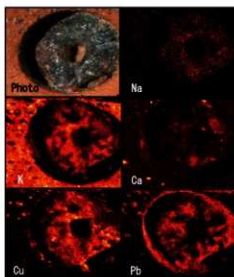
蛍光X線元素マッピング (No. 21)
