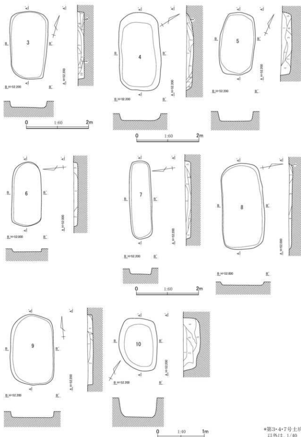
第689图 第3~10号土坑平面·断面图(1)
