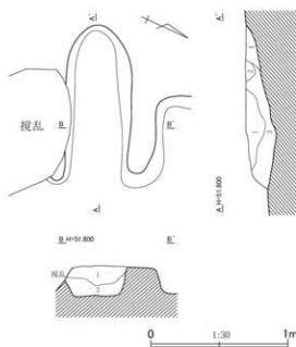
第660図 第309号住居跡平面・断面図
