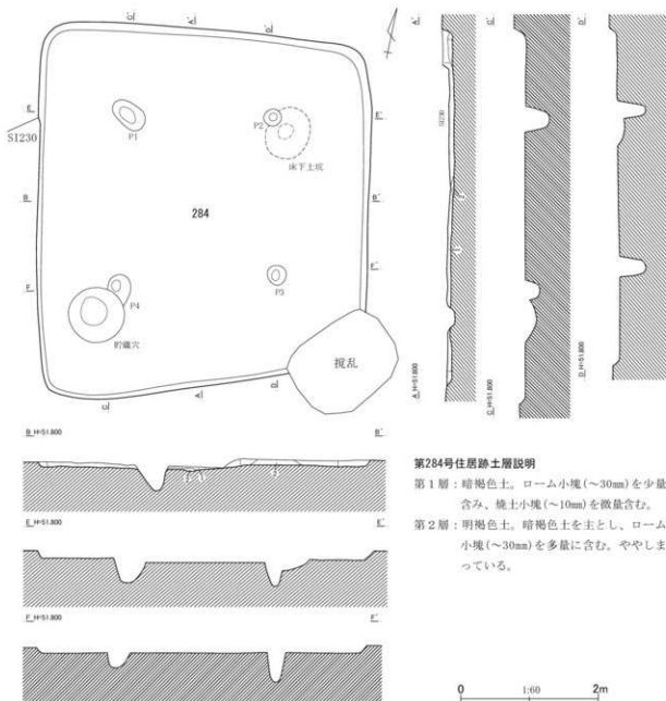
第609図 第284号住居跡平面・断面図（1）
