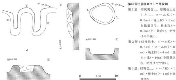
第163図 第86号住居跡平面・断面図（2）
