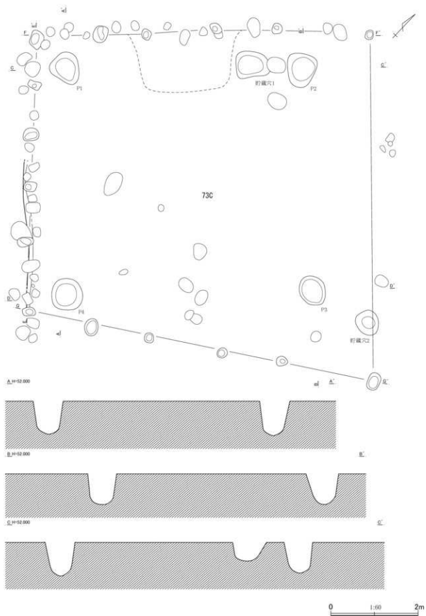
第133图 第73C号住居跡平面・断面图(1)
