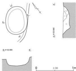
第191図 第101号住居跡平面・断面図(2)
