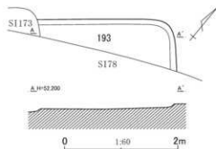
第403図 第193号住居跡平面・断面図
