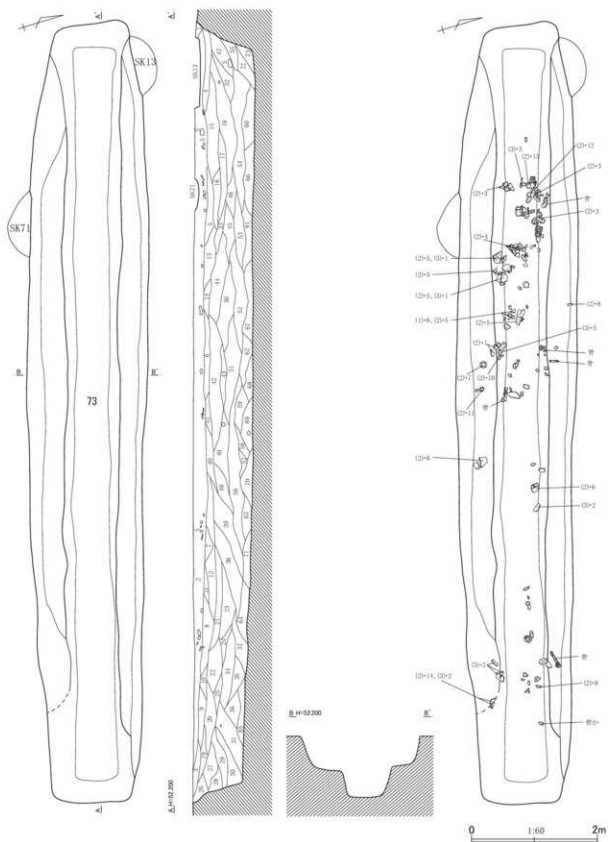
第705图 第73号土坑平面·断面图(1)
