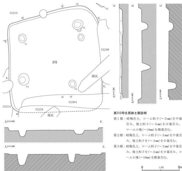
第671図 第315号住居跡平面・断面図
