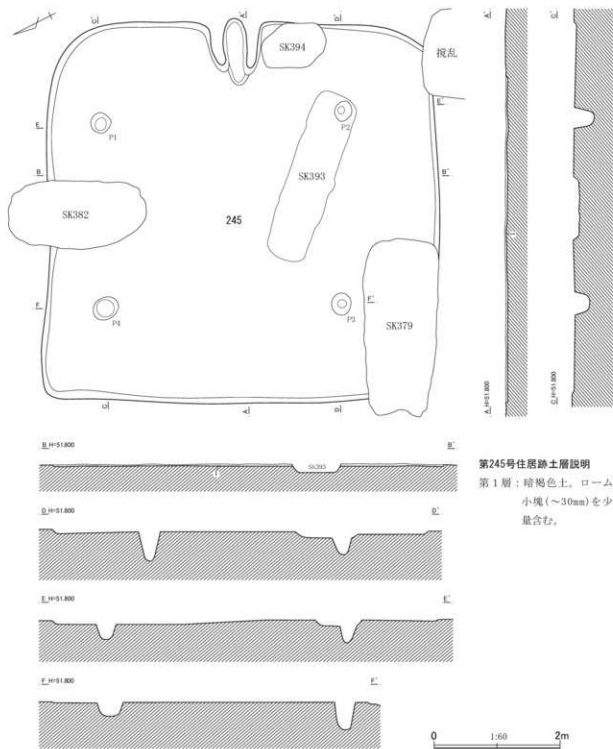
第520図 第245号住居跡平面・断面図（2）
