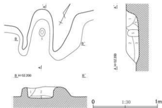
第369図 第176号住居跡平面・断面図(1)
