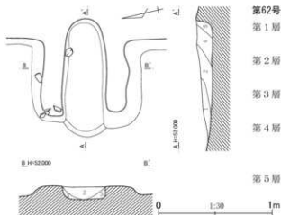
第98図 第62号住居跡平面・断面図
