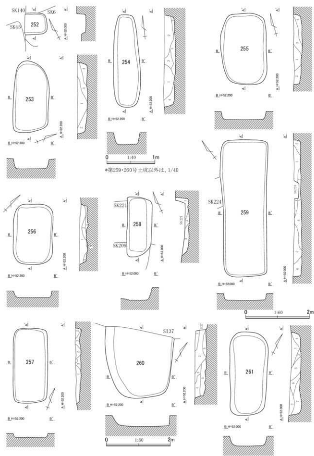
第746图 第252~261号土坑平面·断面图(1)
