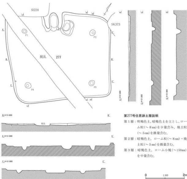
第592図 第277号住居跡平面・断面図(1)
