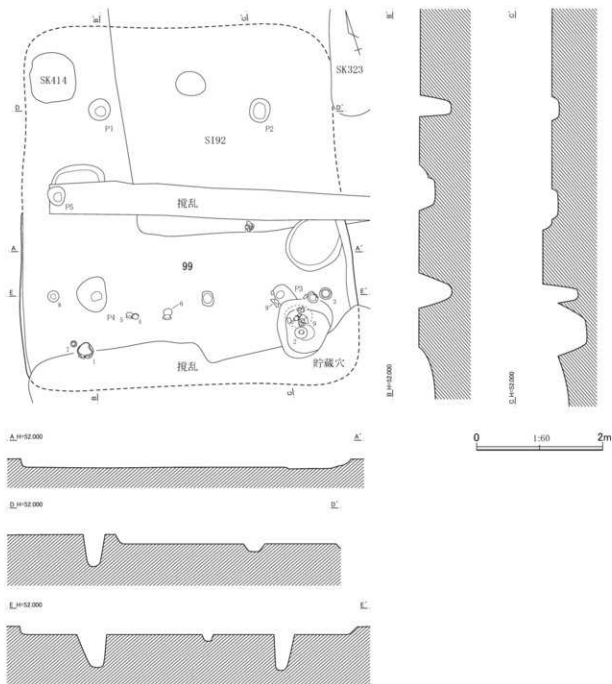
第184図 第99号住居跡平面・断面図(1)
