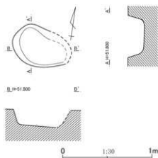
第129図 第73A号住居跡平面・断面図(3)
