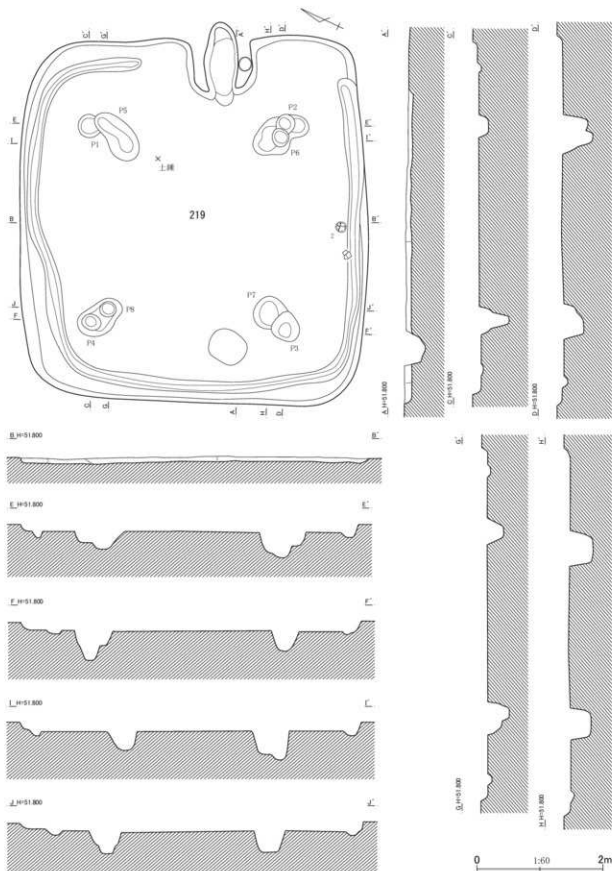
第456图 第219号住居跡平面・断面图(1)
