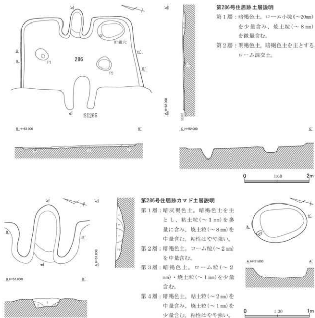
第614図 第286号住居跡平面・断面図
