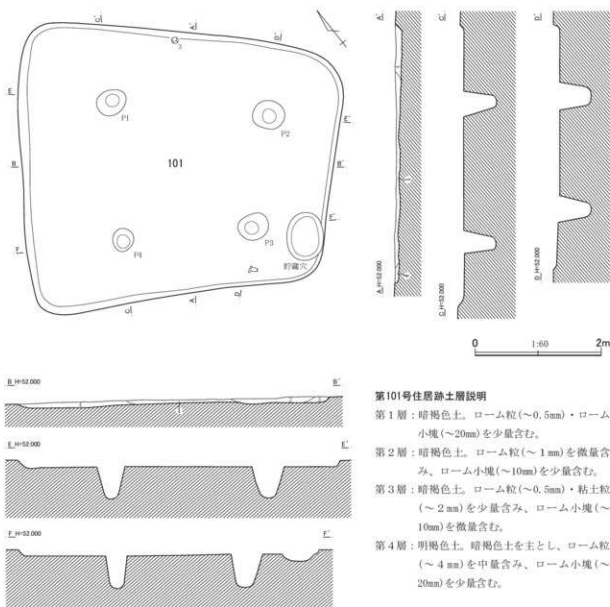
第190図 第101号住居跡平面・断面図(1)
