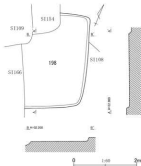
第410図 第198号住居跡平面・断面図
