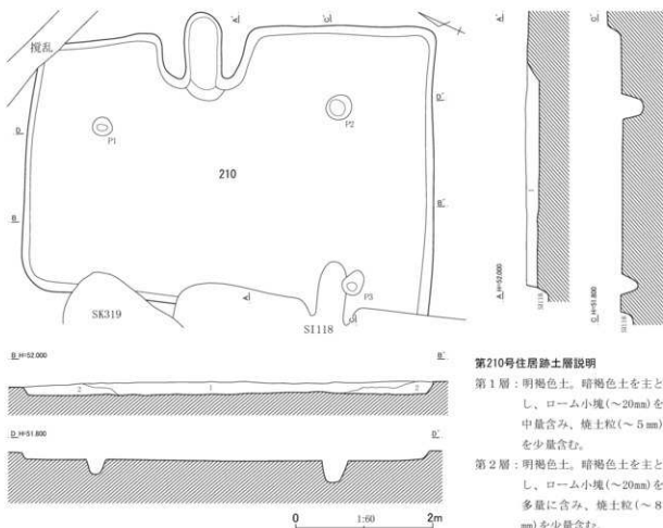
第436図 第210号住居跡平面・断面図(1)
