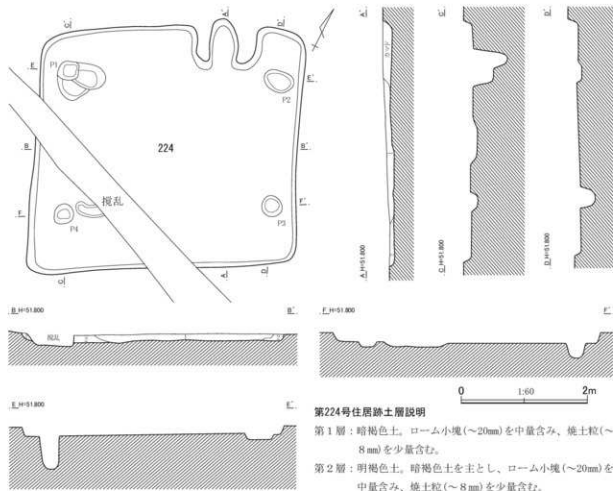
第469図 第224号住居跡平面・断面図(1)
