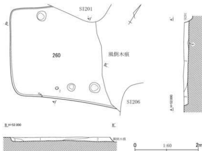
第552図 第260号住居跡平面・断面図
