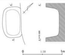
第676図 第318号住居跡平面・断面図(2)
