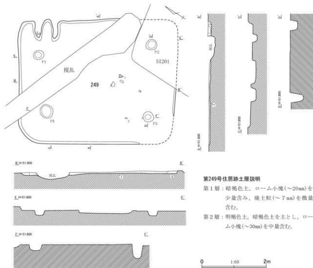
第529図 第249号住居跡平面・断面図(2)
