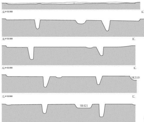
第429図 第207号住居跡平面・断面図（1）
