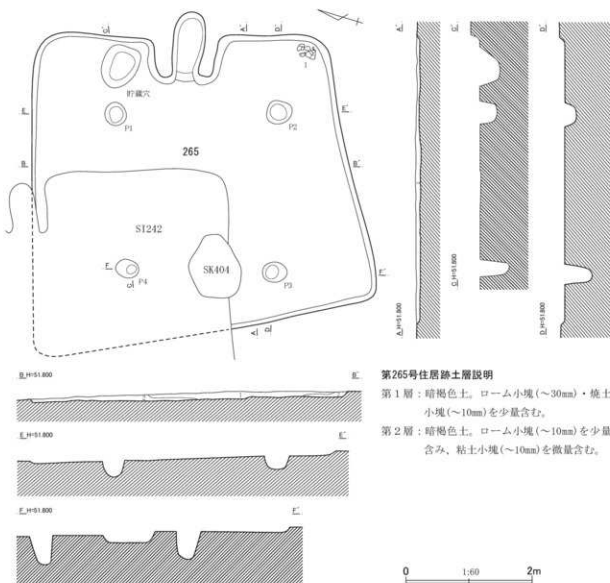
第563図 第265号住居跡平面・断面図(1)
