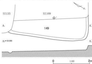
第314図 第149号住居跡平面・断面図
