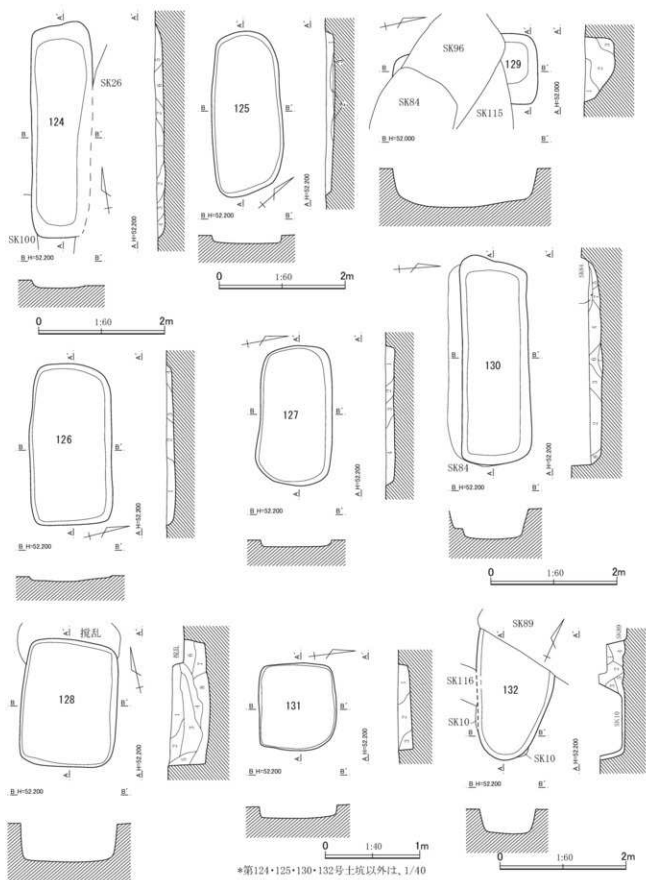
第720图 第124~132号土坑平面·断面图(1)
