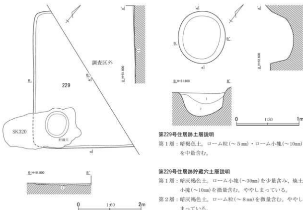
第480図 第229号住居跡平面・断面図
