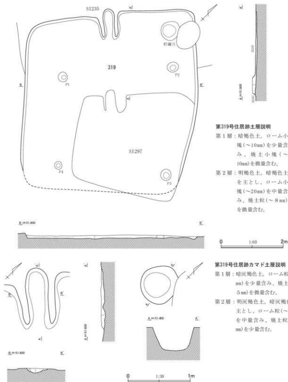
第678図 第319号住居跡平面・断面図
