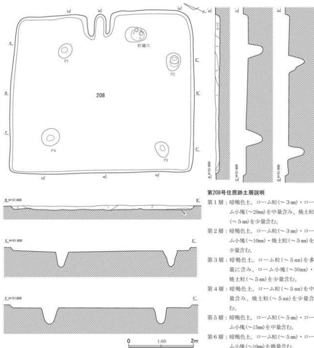
第432図 第208号住居跡平面・断面図(1)
