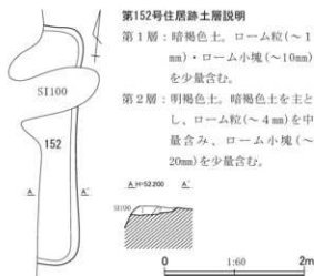
第321図 第152号住居跡平面・断面図
