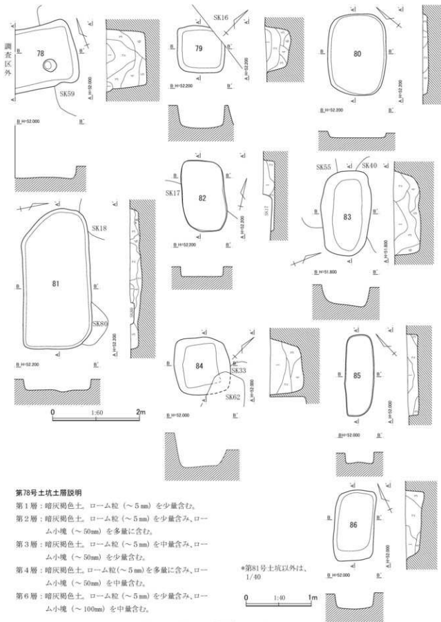
第709図 第78～86号土坑平面・断面図（1）
