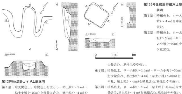
第198図 第103号住居跡平面・断面図(2)
