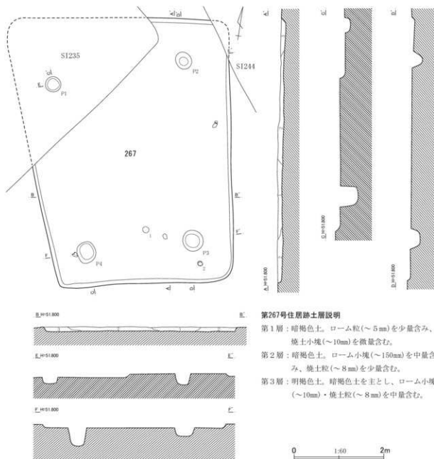
第568図 第267号住居跡平面・断面図
