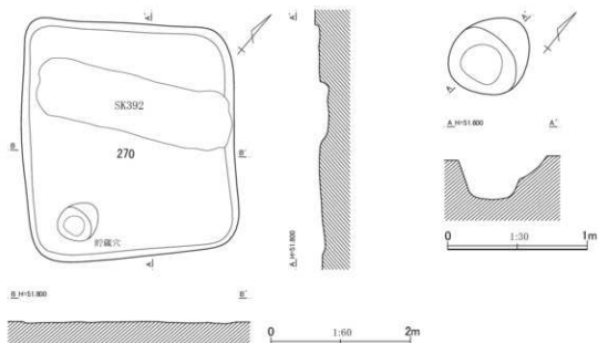
第574図 第269号住居跡平面・断面図
