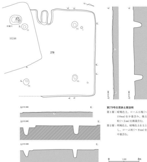
第597図 第279号住居跡平面・断面図（1）
