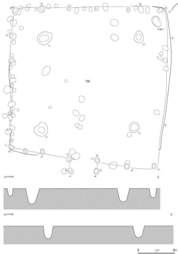
第127图 第73A号住居跡平面・断面图(1)
