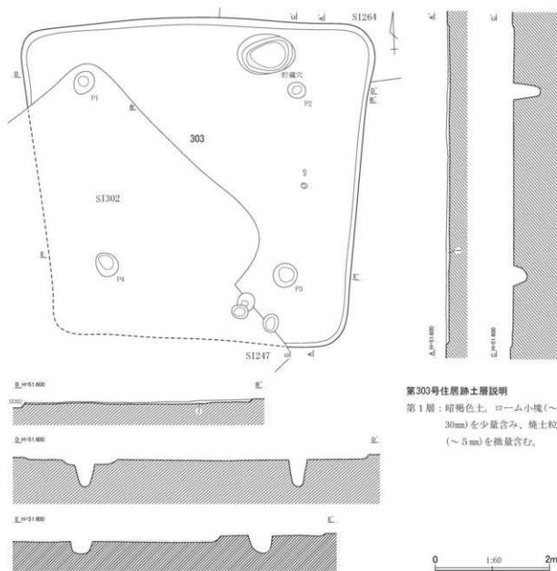
第647図 第303号住居跡平面・断面図(1)
