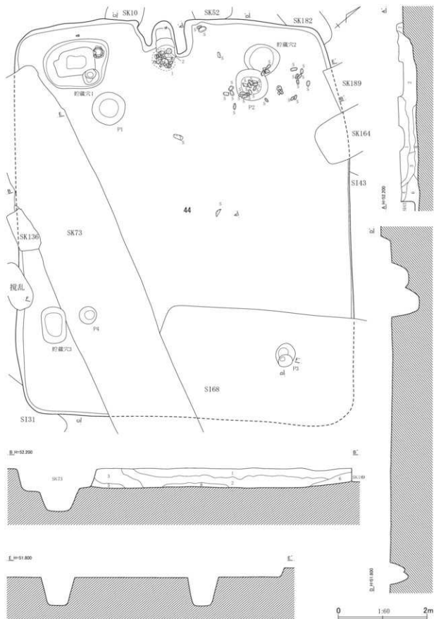
第46図 第44号住居跡平面・断面図(1)
