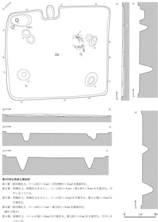
第493図 第235号住居跡平面・断面図(1)
