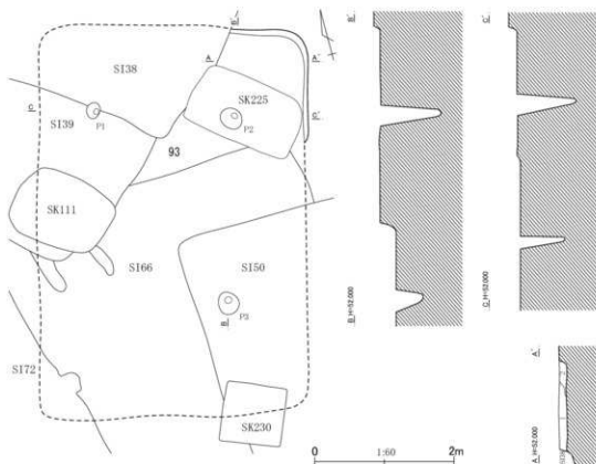
第176図 第93号住居跡平面・断面図(2)
