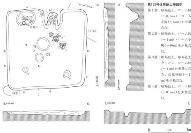
第275図 第133号住居跡平面・断面図（1）
