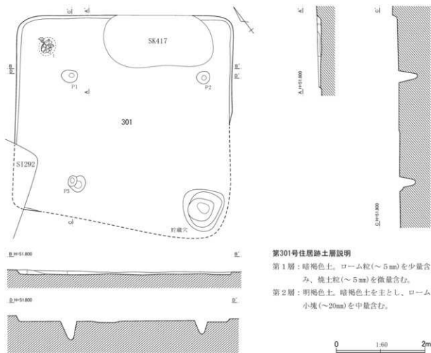
第642図 第301号住居跡平面・断面図（2）
