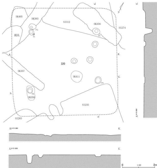
第680図 第320号住居跡平面・断面図
