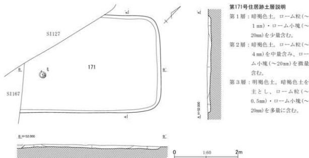
第362図 第171号住居跡平面・断面図
