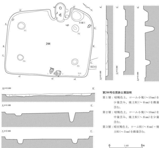
第516図 第244号住居跡平面・断面図(1)
