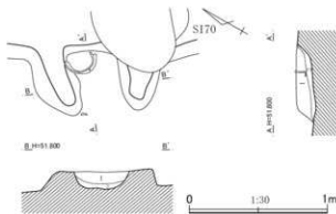
第158図 第84号住居跡平面・断面図
