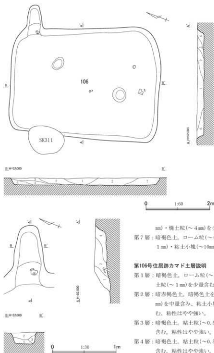
第205図 第106号住居跡平面・断面図
