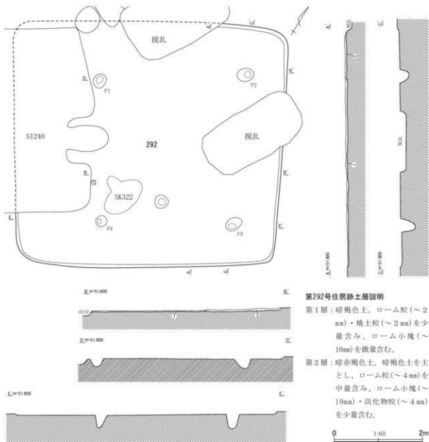
第625図 第292号住居跡平面・断面図
