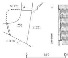
第488図 第233号住居跡平面・断面図
