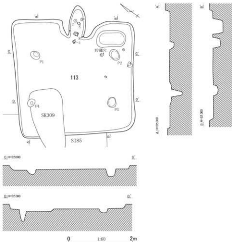
第224図 第113号住居跡平面・断面図(1)
