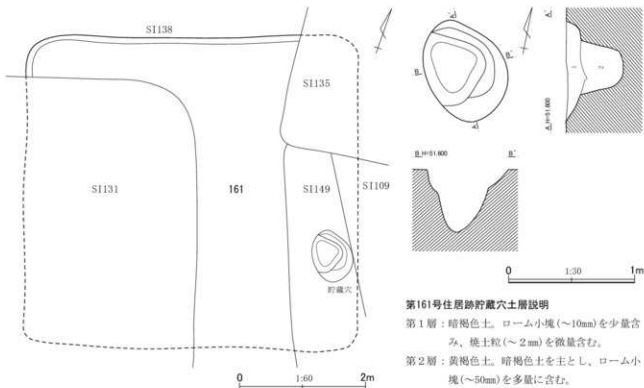
第340図 第161号住居跡平面・断面図
