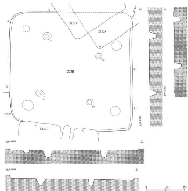
第579图 第272号住居跡平面・断面图
