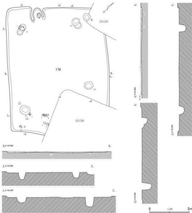
第374図 第178号住居跡平面・断面図(2)
