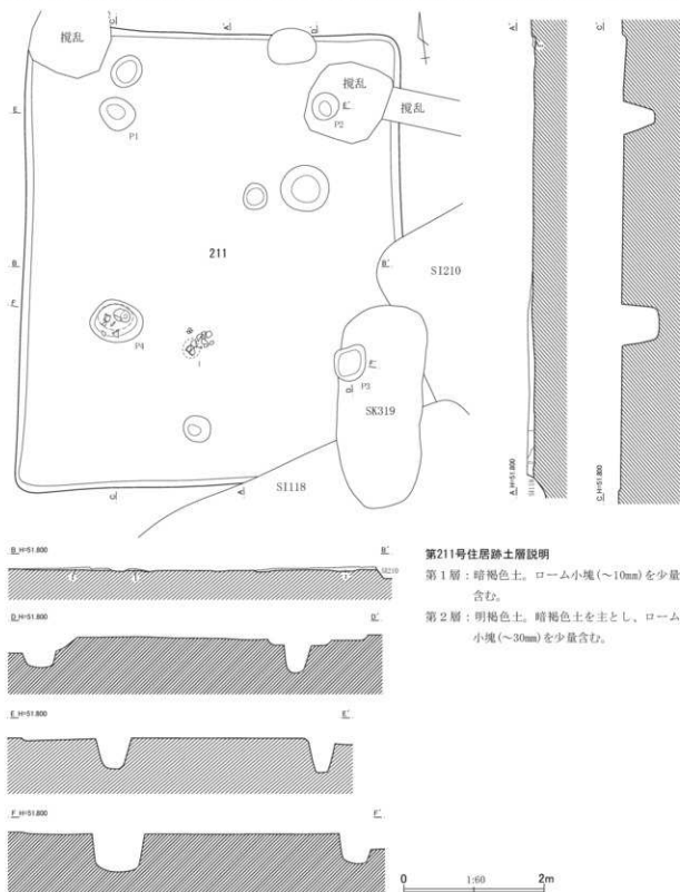
第439図 第211号住居跡平面・断面図
