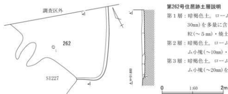
第556図 第262号住居跡平面・断面図
