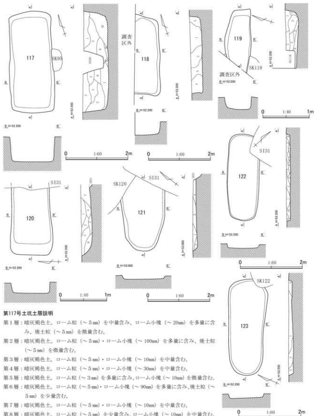
第718図 第117～123号土坑平面・断面図（1）
