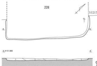
第478図 第228号住居跡平面・断面図
