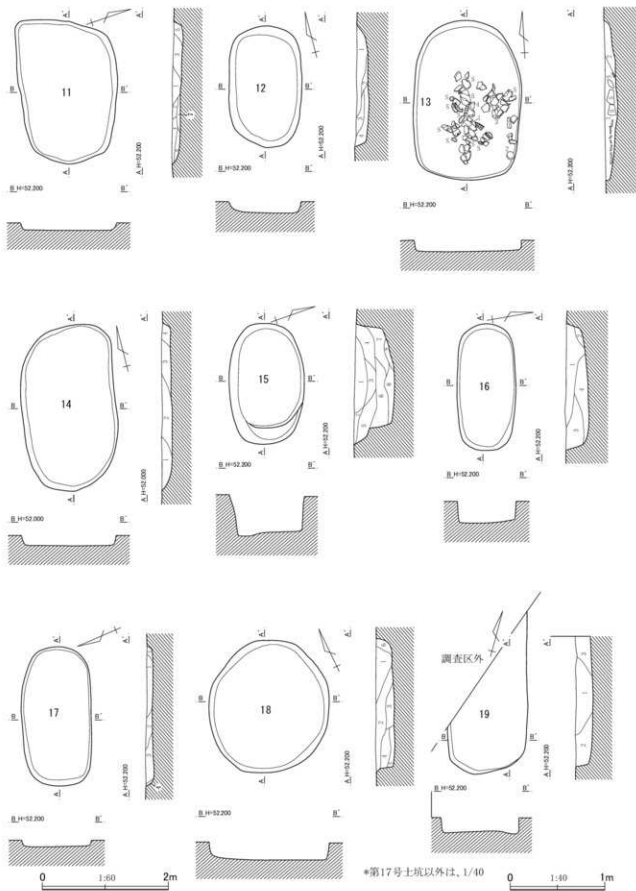
第691图 第11~19号土坑平面·断面图(1)
