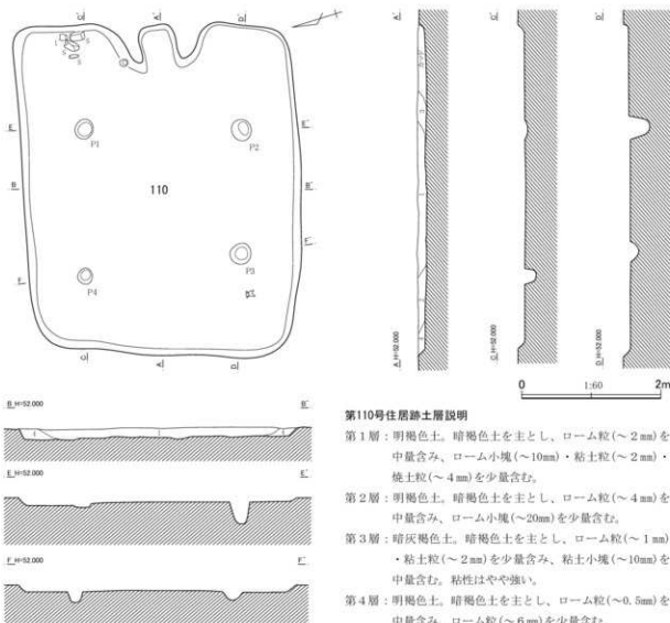
第216図 第110号住居跡平面・断面図(1)
