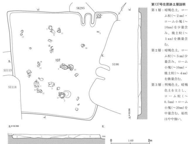
第285図 第137号住居跡平面・断面図(1)
