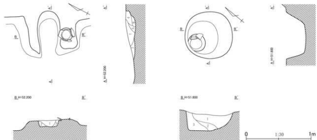
第77図 第55号住居跡平面・断面図(1)
