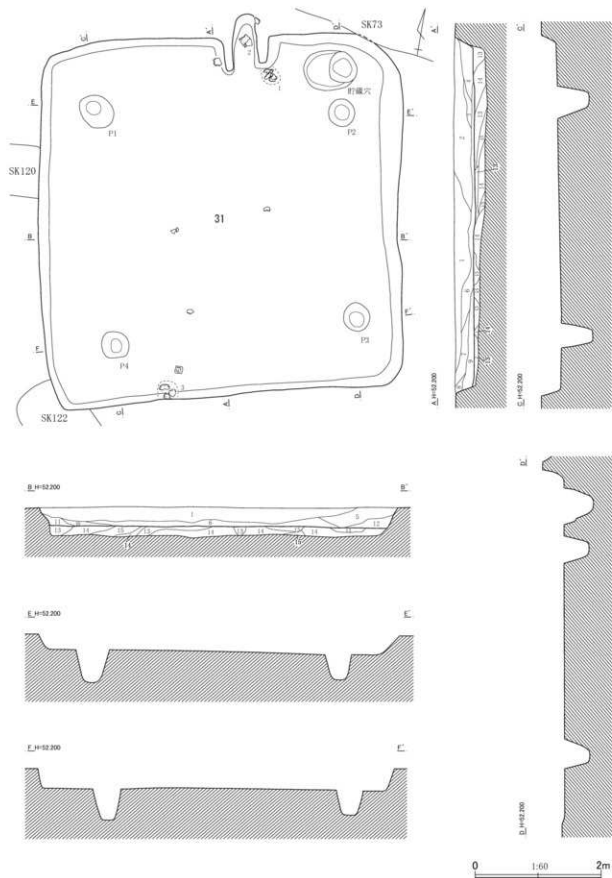
第10図 第31号住居跡平面・断面図(1)
