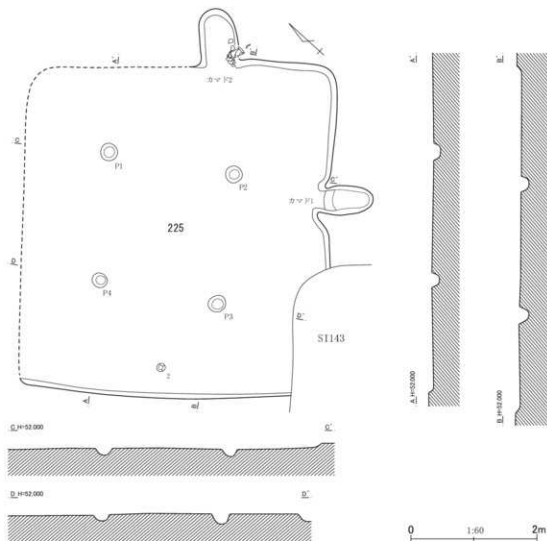
第471図 第225号住居跡平面・断面図(1)
