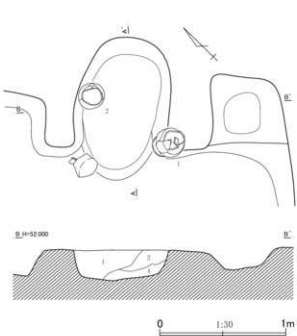
第54図 第47号住居跡平面・断面図(2)
