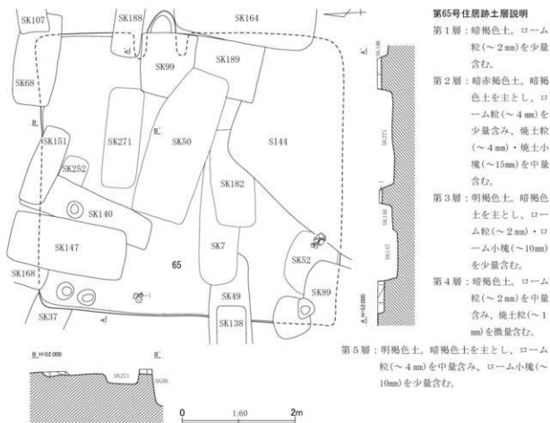
第105図 第65号住居跡平面・断面図（1）
