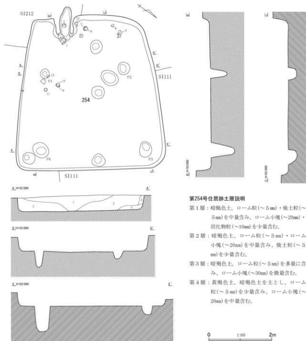
第539図 第254号住居跡平面・断面図（1）
