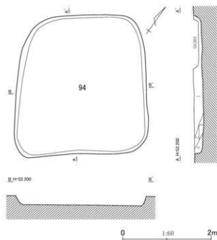
第178図 第94号住居跡平面・断面図
