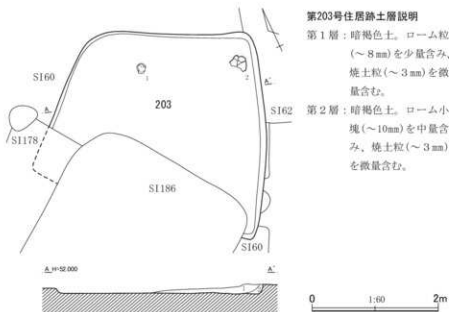
第419図 第203号住居跡平面・断面図
