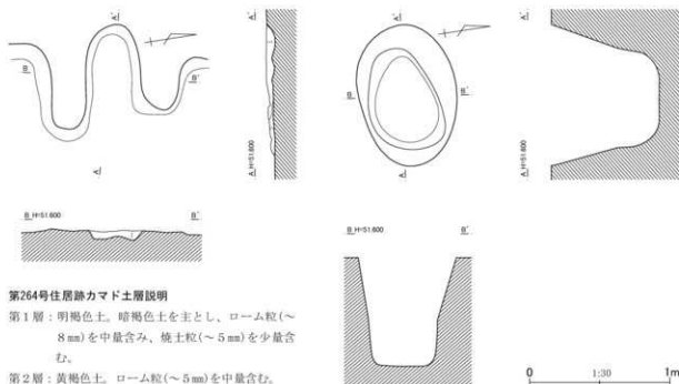
第560図 第264号住居跡平面・断面図(1)
