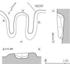
第286図 第137号住居跡平面・断面図(2)
