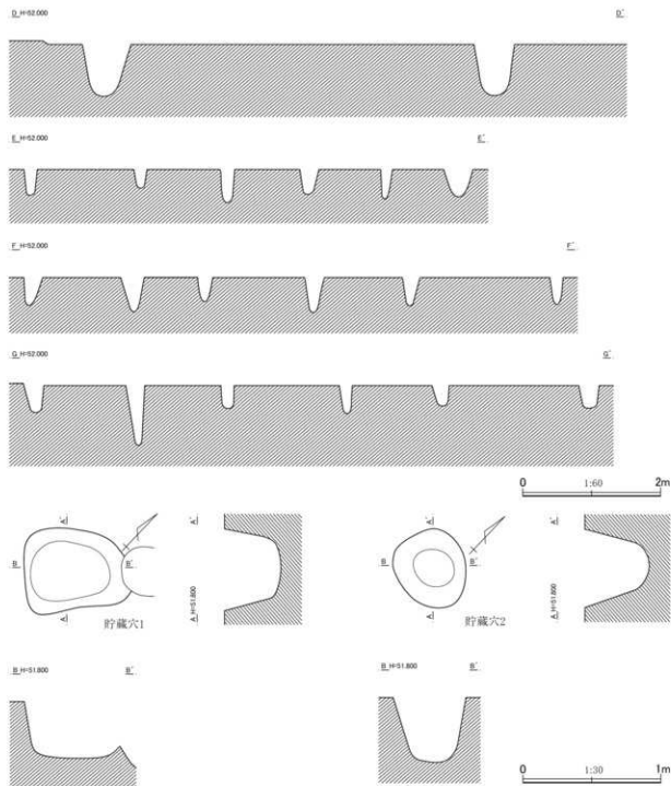
第134図 第730号住居跡平面・断面図(2)
