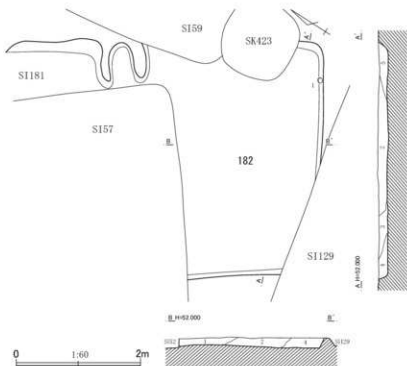
第382図 第182号住居跡平面・断面図(1)
