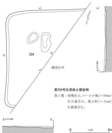
第421図 第204号住居跡平面・断面図
