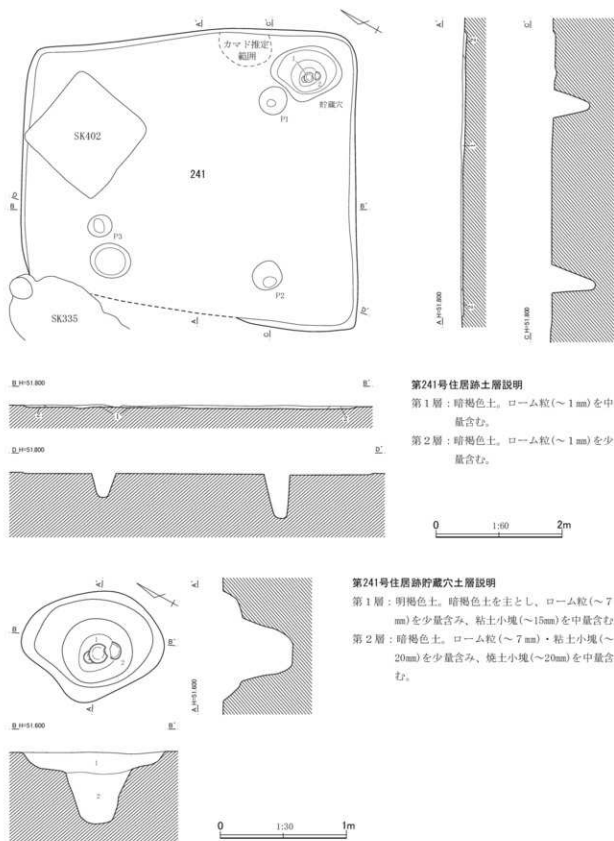
第508図 第241号住居跡平面・断面図
