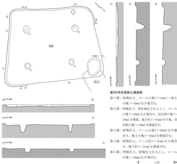
第644図 第302号住居跡平面・断面図(1)
