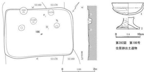
第391図 第186号住居跡平面・断面図
