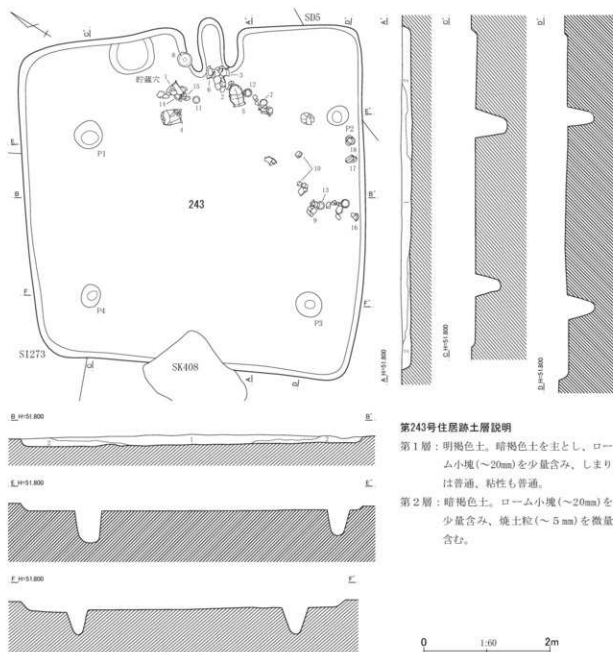
第513図 第243号住居跡平面・断面図(1)
