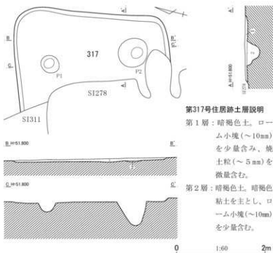
第674図 第317号住居跡平面・断面図
