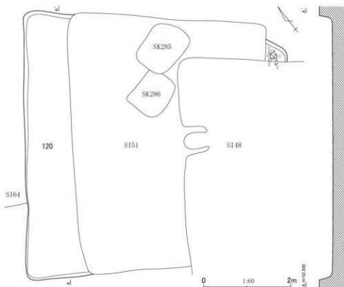
第246図 第120号住居跡平面・断面図
