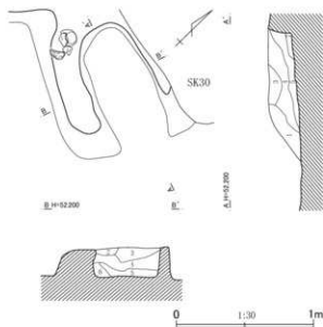
第113図 第67号住居跡平面・断面図(2)
