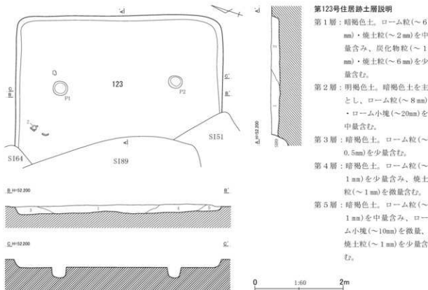
第253図 第123号住居跡平面・断面図
