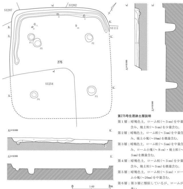
第586図 第275号住居跡平面・断面図
