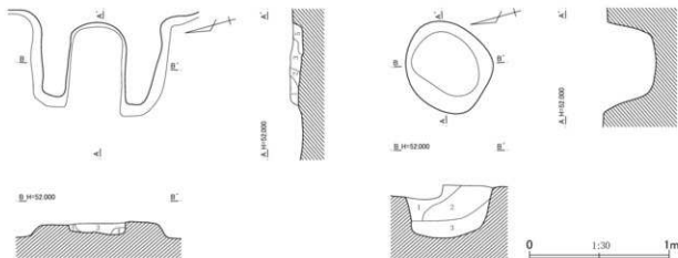
第121図 第70号住居跡平面・断面図(1)
