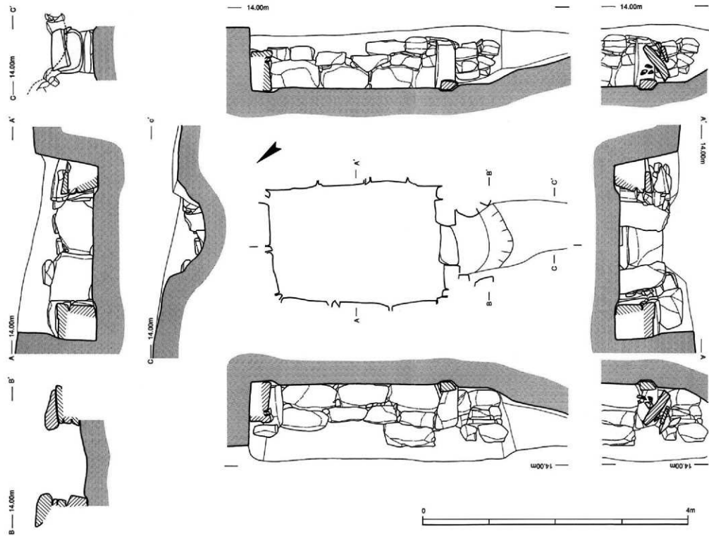
第30图 大浦古墳群10号墳石室実測図 (S=1/40)
