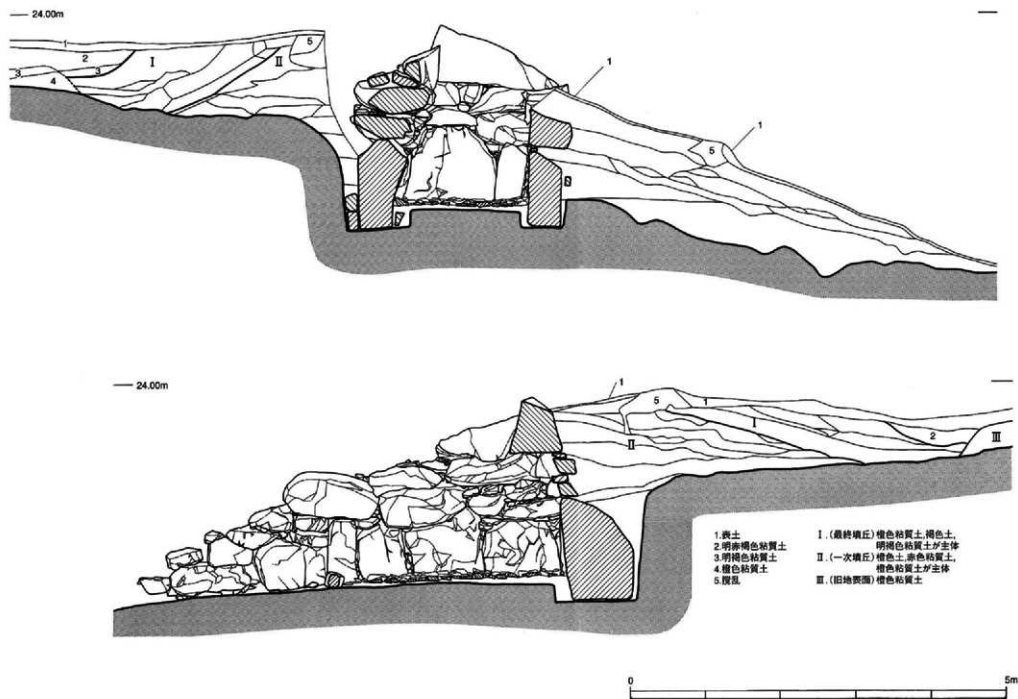
第3图 浦边古坟群1号墳填丘土层断面图 (S=1/50)
