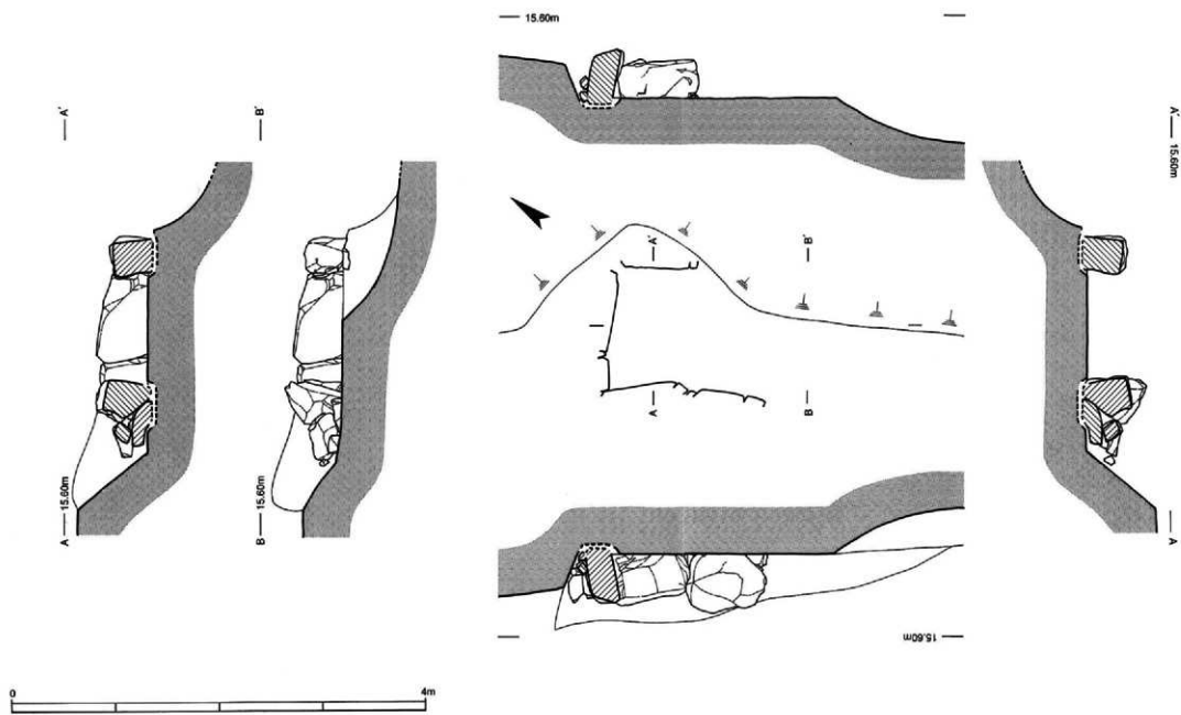
第46图 梅ヶ崎古墳群5号埴石室実測図 (S=1/40)
