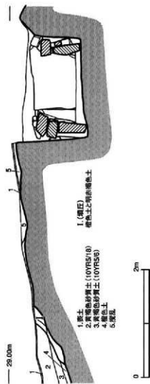
第12图 大浦古坟群2号坟丘土层断面图 (S=1/50)
