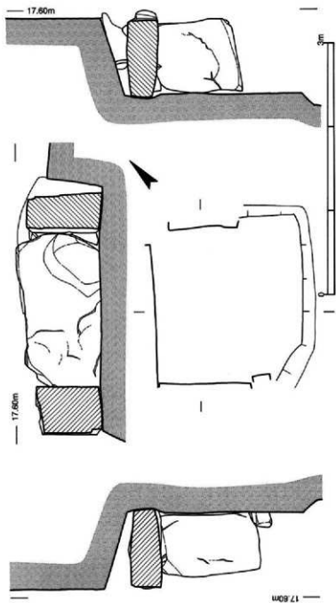
第20図 大浦古墳群6号墳石室実測図 (S=1/40)
