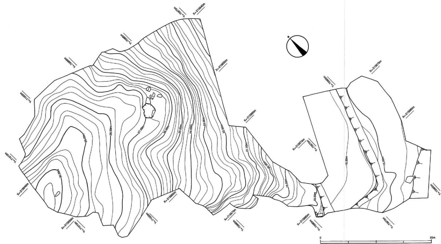
第8图 大浦古墳群I地区調査前地形測量図 (S=1/200)
