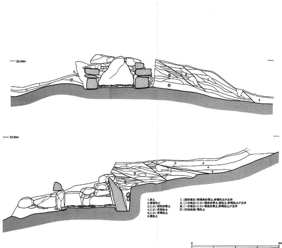
第18図 大浦古墳群5号墳積丘土層断面図 (S=1/50)
