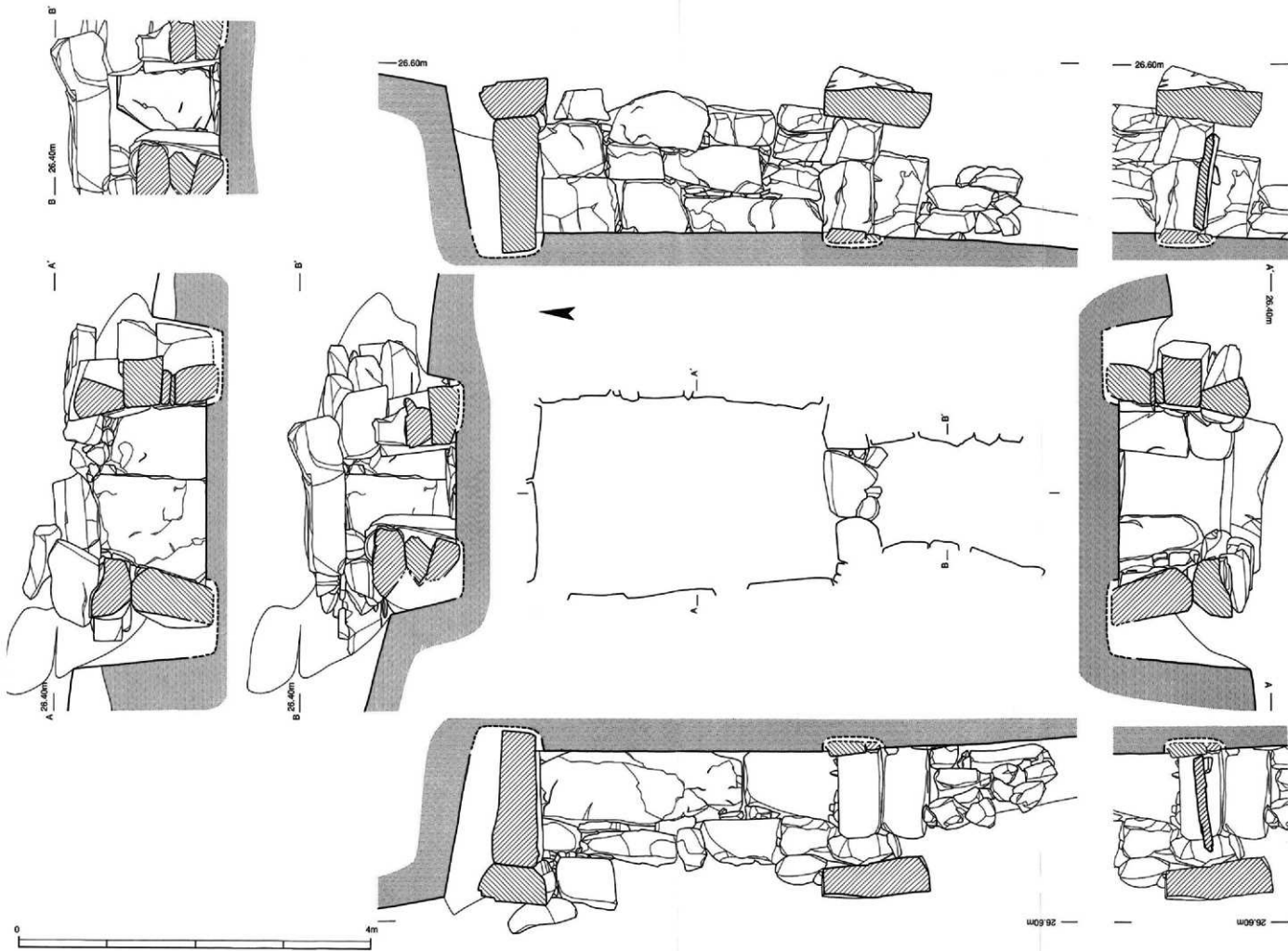
第17图 大浦古墳群4号墳石室实测图 (S=1/40)
