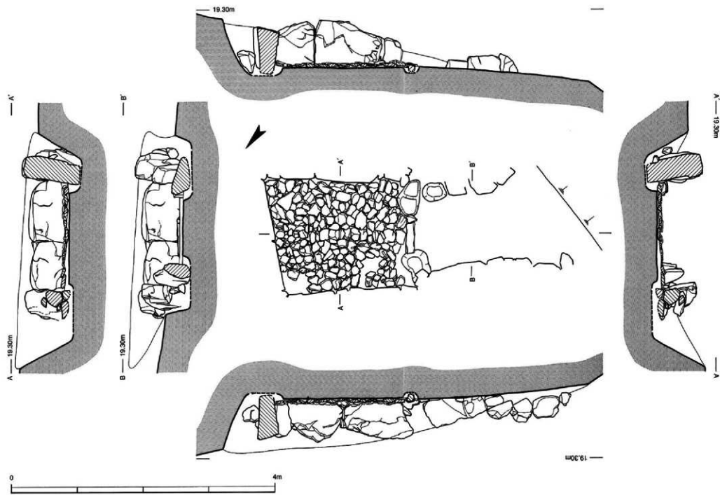
第42図 梅ヶ崎古墳群3号墳石室実測図 (S=1/40)
