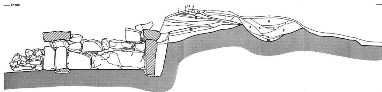
第16図 大浦古墳群4号墳丘土層断面図 (S=1/50)
