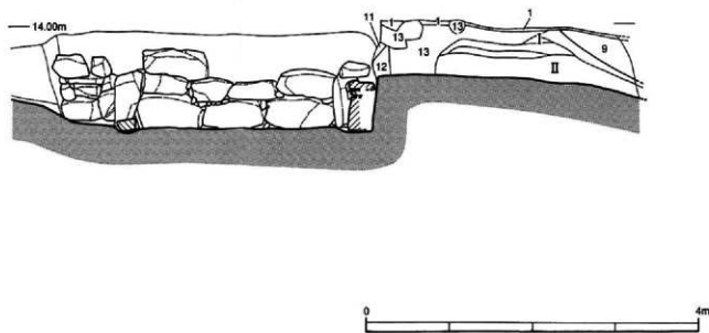
第29図 大浦古墳群10号墳填丘土層断面図 (S=1/50)
