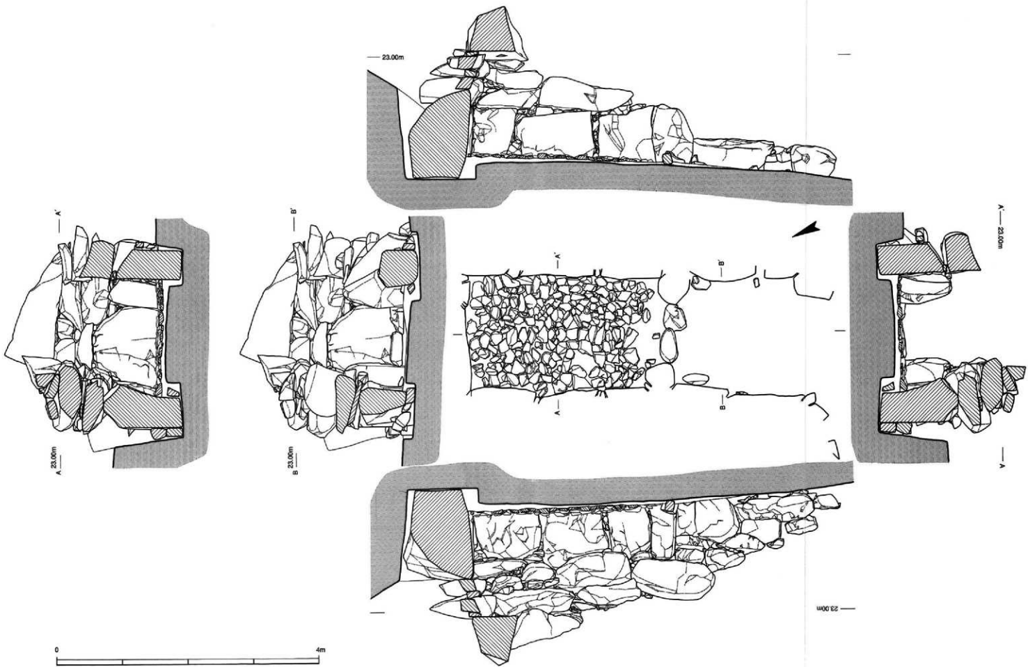
第4图 浦边古墳群1号墳石室実測図 (S=1/40)
