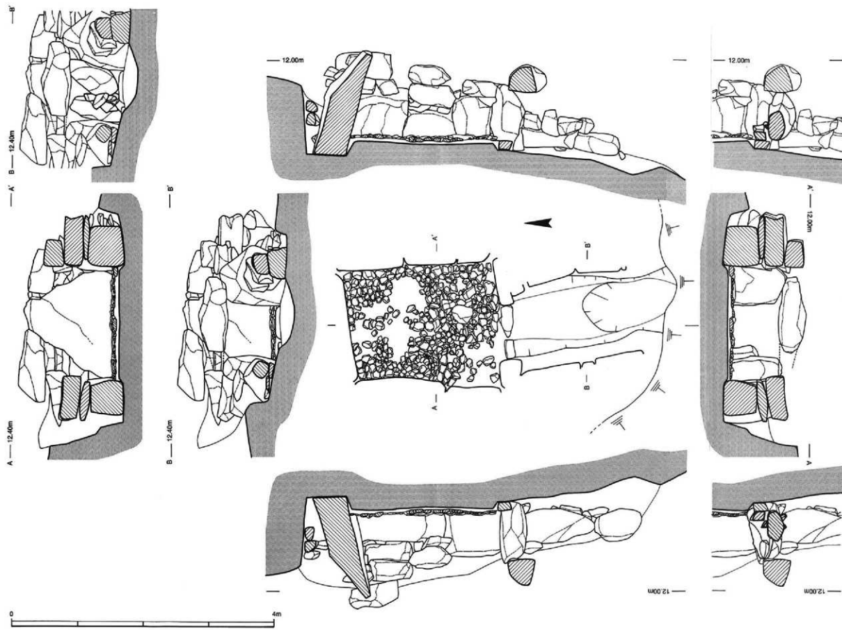
第19図 大浦古墳群5号墳石室実測図 (S=1/40)
