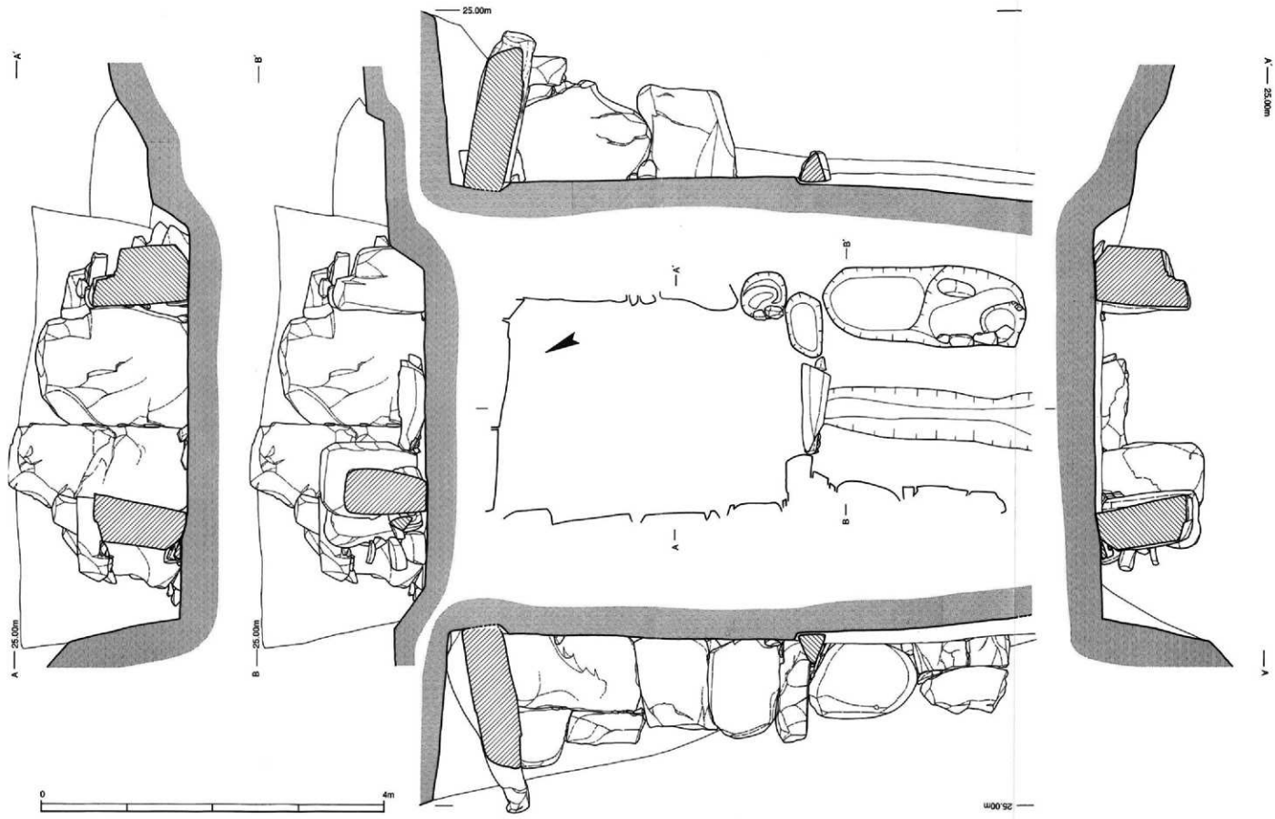
第6图 浦边古墳群2号墳石室実測図 (S=1/40)
