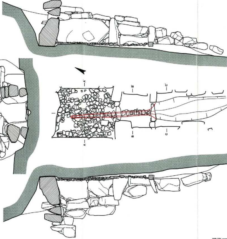
第34回 大浦古墳群12号墳石室実測図 (S=1/40)
