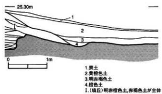
第7图 浦边古坟群3号填丘土層断面図 (S=1/50)
