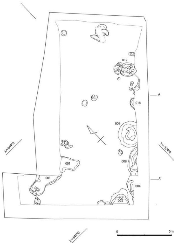
图 5. 遺構配置図 (1/100)
