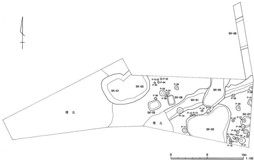
图 4 遺跡全体図
