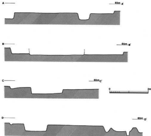
第11図 下田遺跡第78、79号住居址断面図
