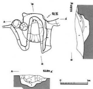
第42図 下田遺跡第133号住居址カマド実測図
