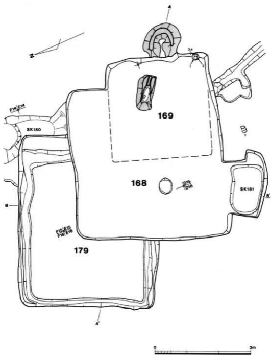
第59図 下田遺跡第168、169、179号住居址夾測図
