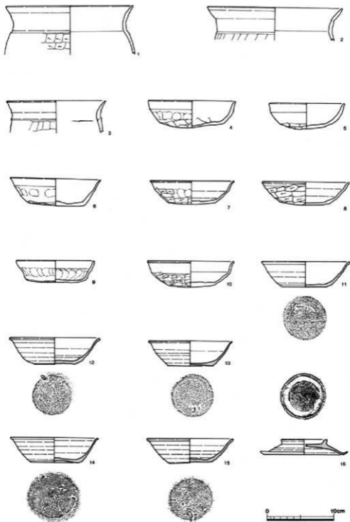
第90圖 元宮遺跡第2号住居址出土遺物実測図(1)
