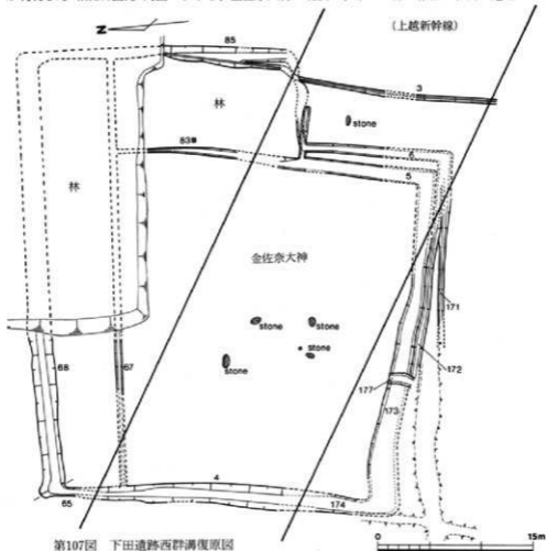
第107図 下田遺跡西群溝復原図
