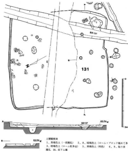
第34図 下田遺跡第131号住居址実測図
