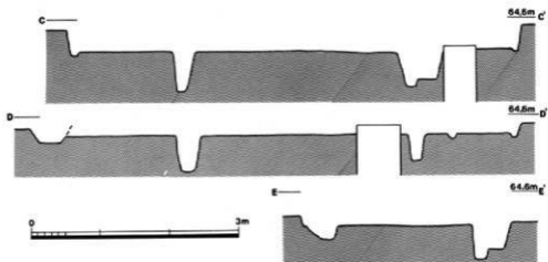
第28図 下田遺跡第122、123号住居址断面図
