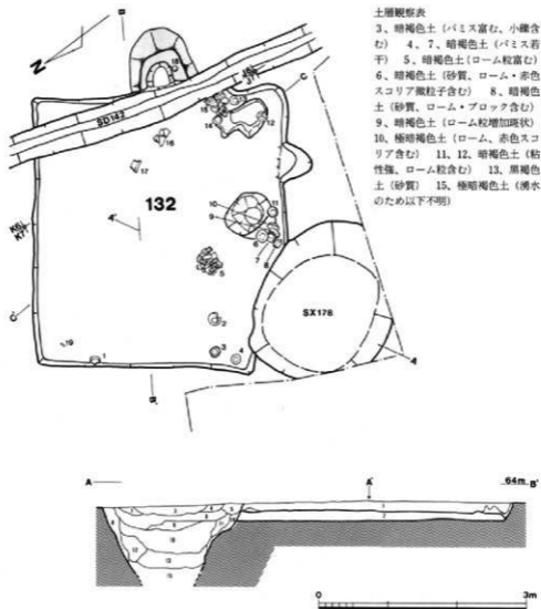
第36図 下田遺跡第132号住居址実測図
