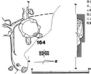
第57図 下田遺跡第164号住居址実測図
