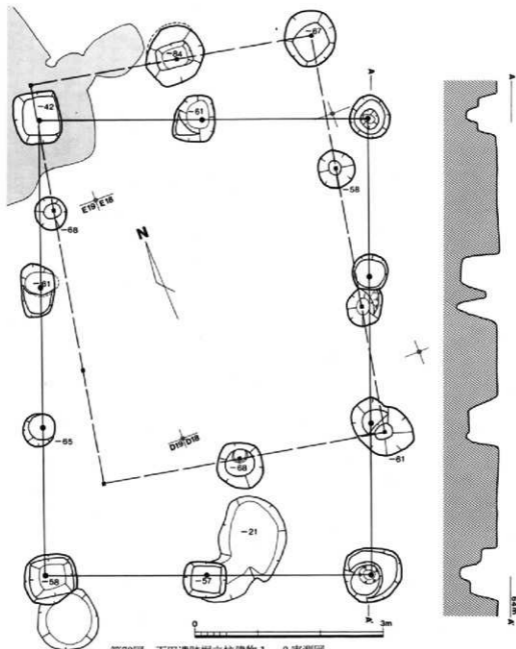
第72図 下田遺跡掘立柱建物 1、2 実測図
