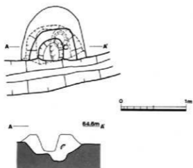
第38図 下田遺跡第132号住居址カマド実測図
