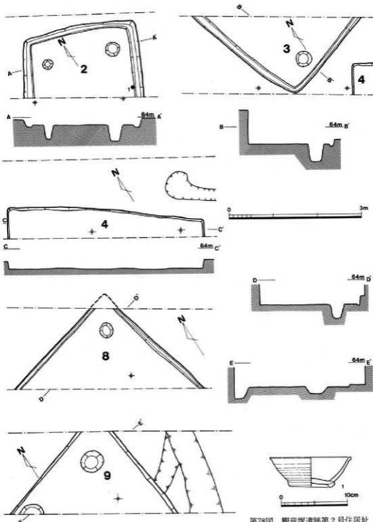
第77图 观音塚遺跡住居址実測図 (第1次調査時)
