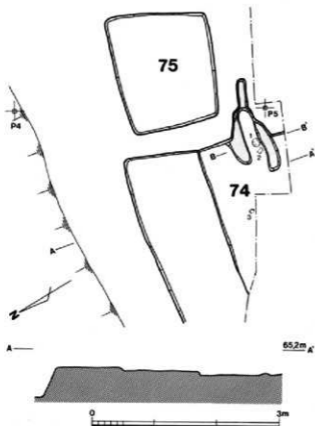
第6図 下田遺跡第74号住居址実測図
