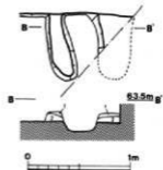
第95図 七色塚遺跡第4号住居址カマド実測図
