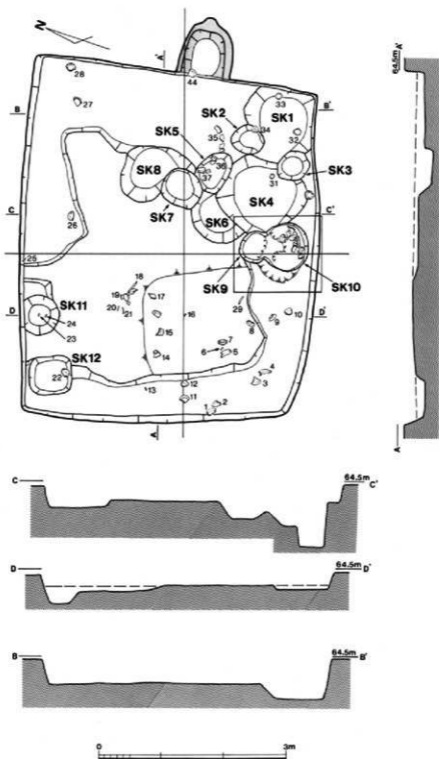
第89圖 元富遺跡第2号住居址実測図
