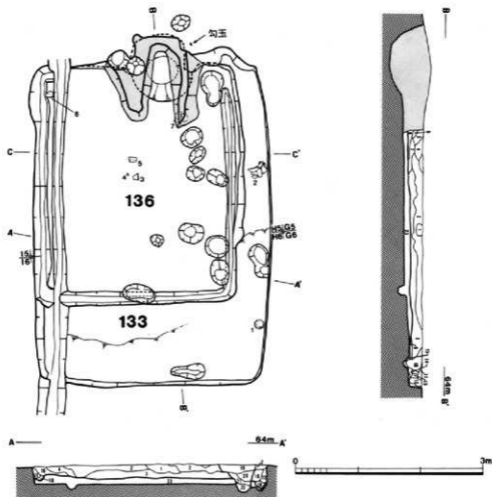
第40回 下田遺跡第133、136号住居址実測図
