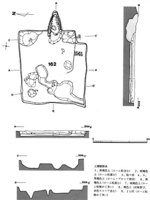
第51図 下田遺跡第162号住居址実測図
