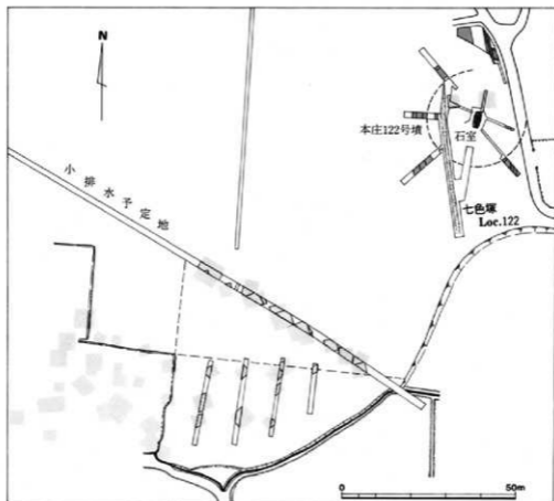
第91図 七色塚遺跡全測図
