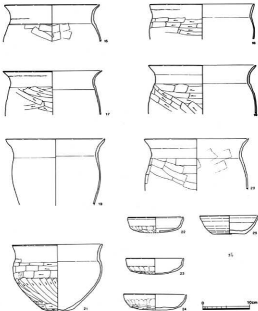
第84図 観音塚遺跡出土遺物実測図(2)
