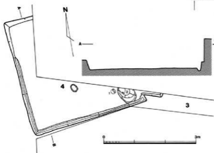
第103図 七色塚遺跡Loc122第3、4、5号住居址実測図
