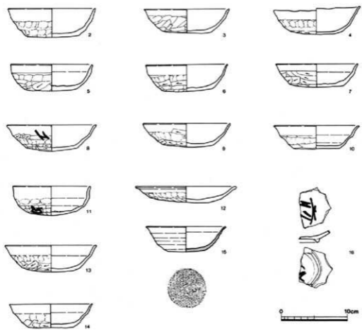
第39图 下田遺跡第132号住居址出土遺物実測図
