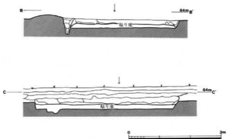
第37図 下田遺跡第132号住居址断面図
