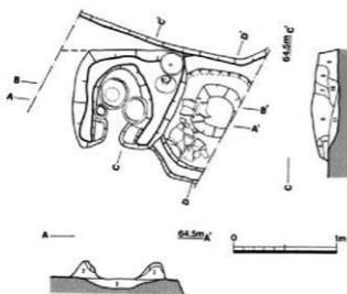
第96図 七色塚遺跡第5A号住居址カマド実測図
