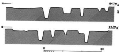
第19図 下田遺跡第93号住居址実測図
