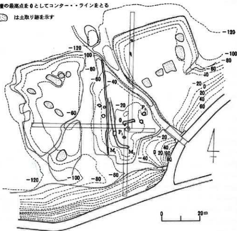
第3図 宝幢寺跡地形異測図
