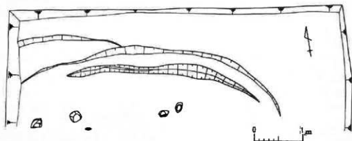
第2図 住居址平面図
