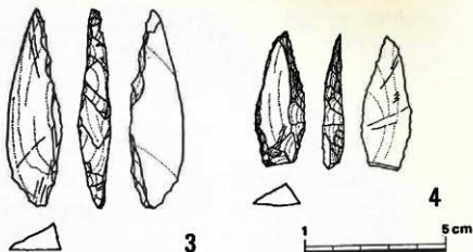
ナイフ形石器実測図
