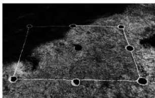
8 第7号掘立柱建物跡
