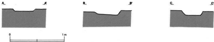
第14図 第1号溝エレベーション
