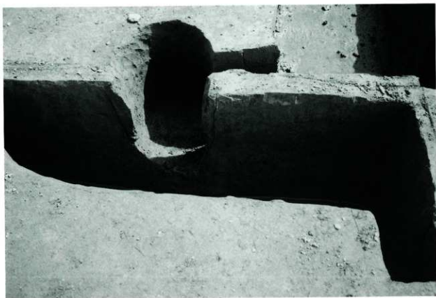
1 第251号住居跡カマド (掘方)
