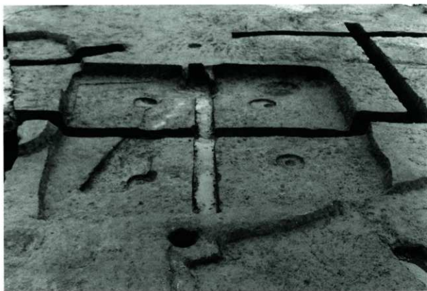
1 第197号住居跡 (柱穴)
