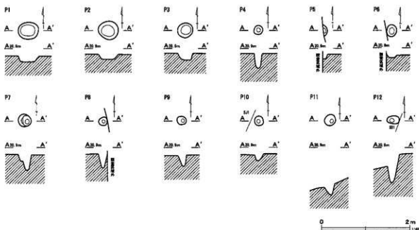
第16図 ビット
