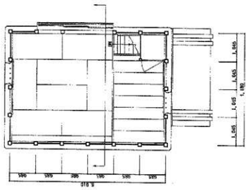
53 修理前 土蔵 2階平面図
