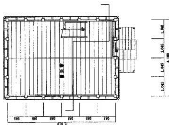
13 竣工 土蔵 1階平面図
