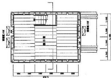
14 竣工 土蔵 2階平面図
