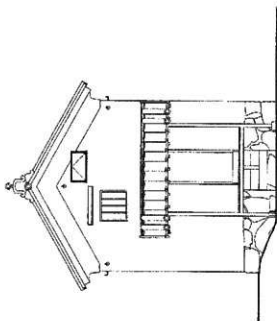
15 竣工 土蔵 正面 (南) 図
