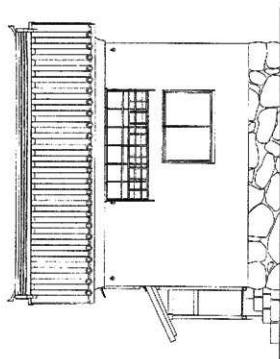
55 修理前 土蔵 東側面図
