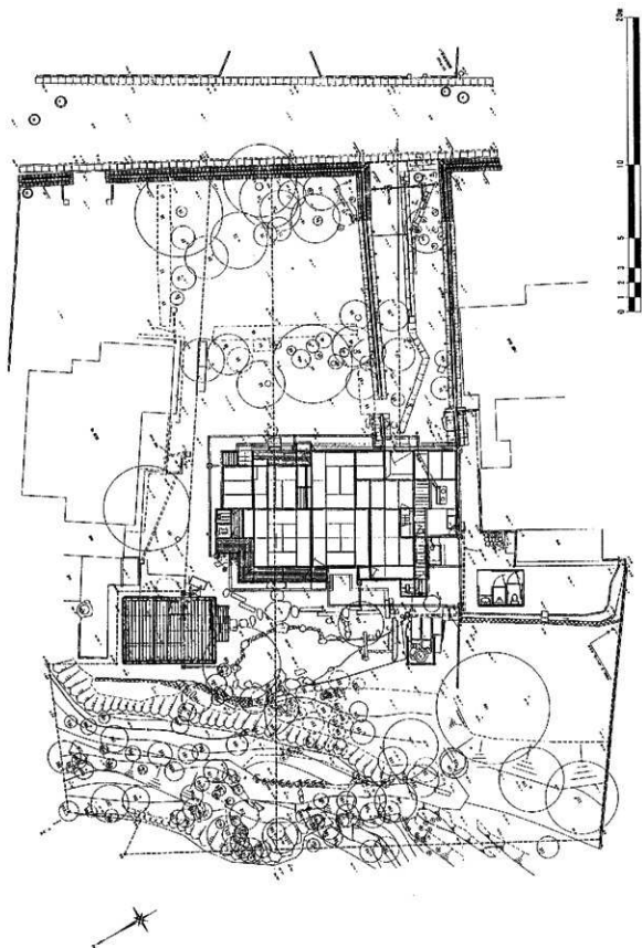
62 修理前 配置図
