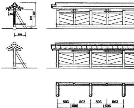
30 竣工 庭板塀一般図 (一般部)
