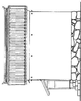
16 竣工 土蔵 裏側面図
