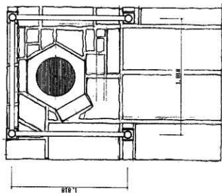
21 竣工 井戸屋形 平面図
