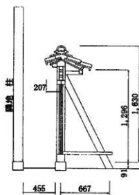
30 竣工 庭板塀一般図 (一般部)
