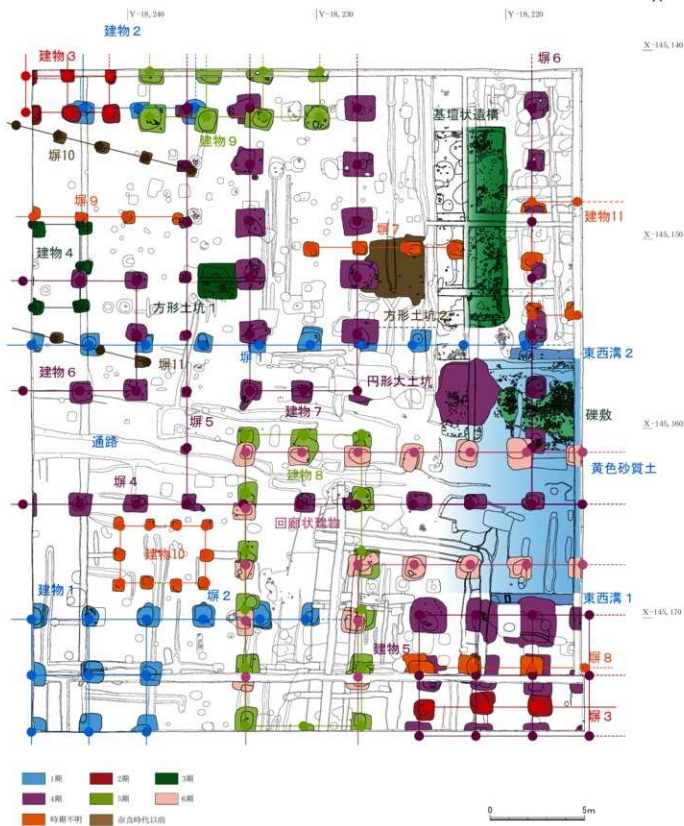
图 3 遺構平面図
