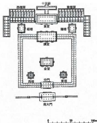
図2 薬師寺伽藍配置図
