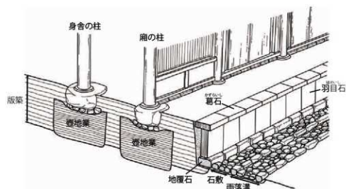
図4 基礎および基礎周辺の模式図
