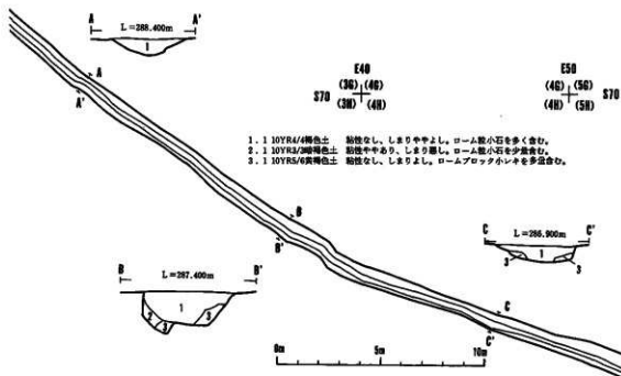
第14図 溝状遺構
