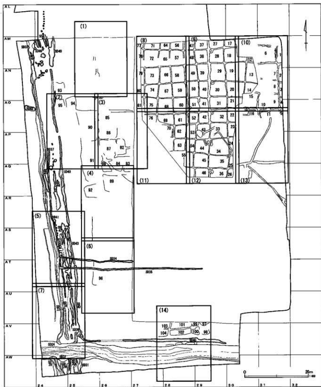
第217图 B区一面水田跡区劃圖
