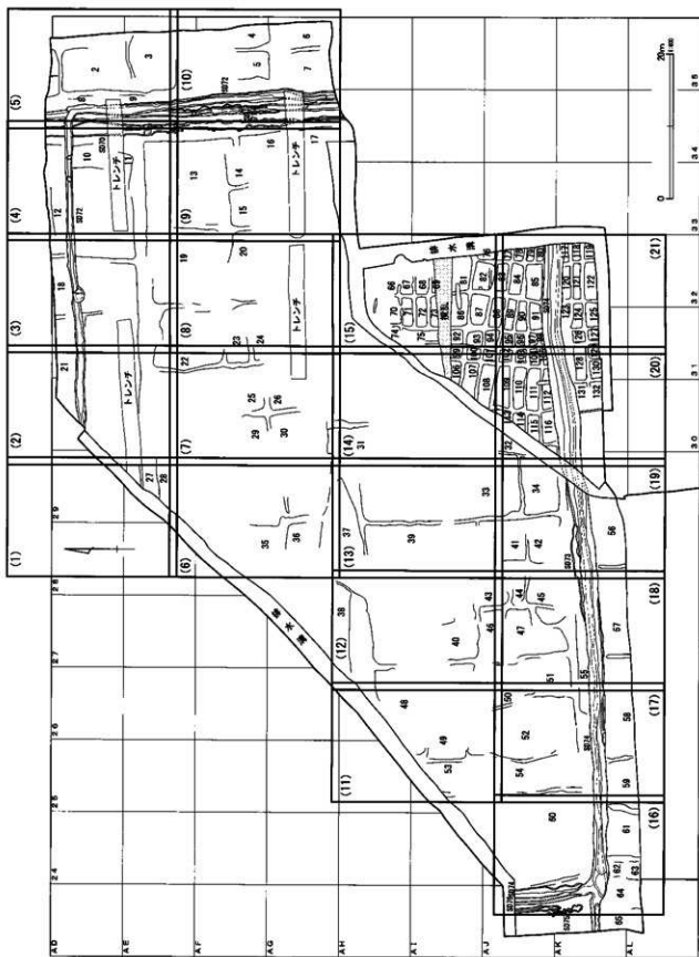
第239図 C区一面水田跡区割図
