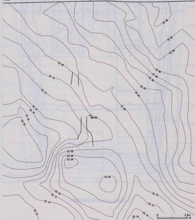
第218图 B区水田跡 (1)
