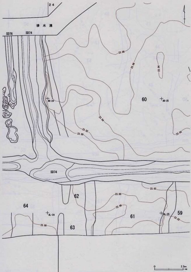
第255図 C区水田跡 (16)
