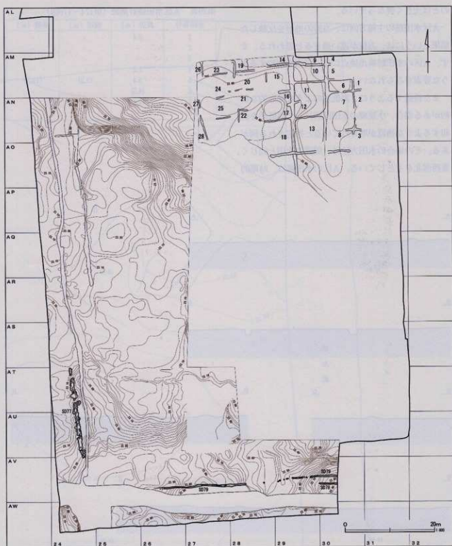
第180图 B区二面水田跡等高线图
