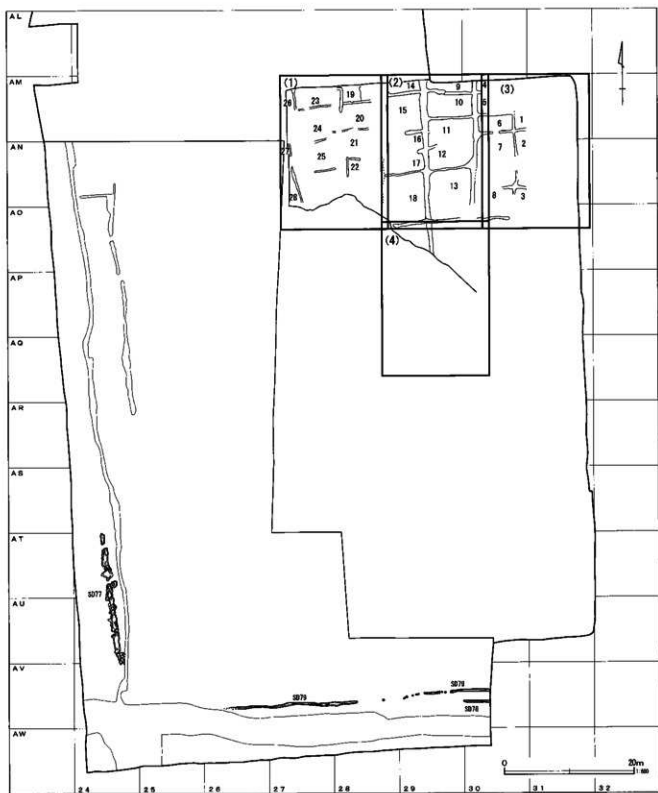
第182图 B区二面水田跡区割图
