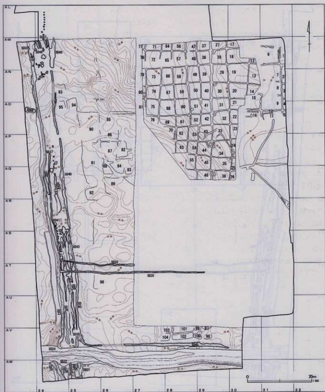
第215图 B区一面水田跡等高線
