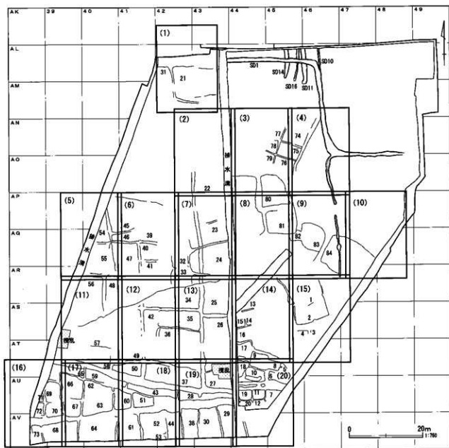
第191図 A区一面水田跡区割図
