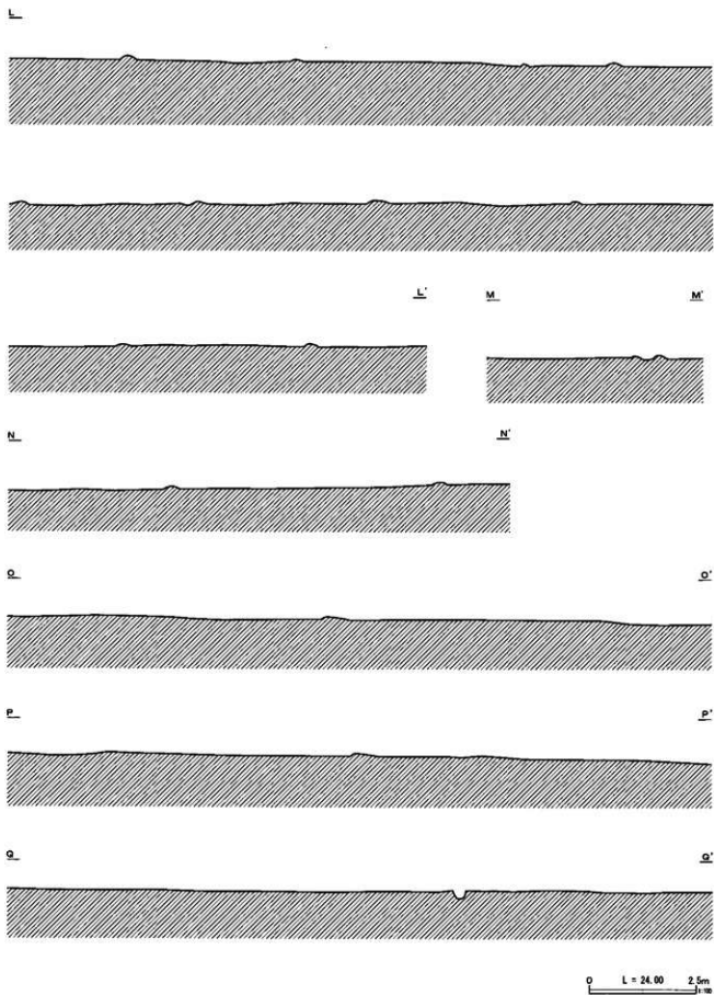
第235図 B区水田跡エレベーション図(4)
