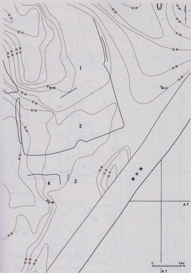
第206团 A区水田跡 (15)
