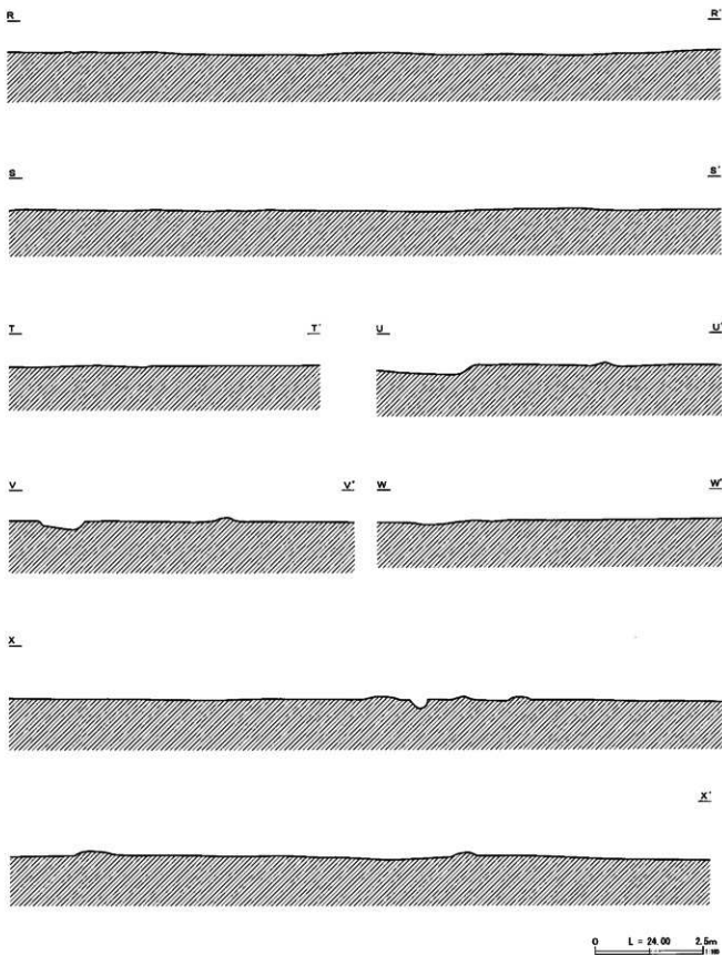
第236図 B区水田跡エレベーション図(5)
