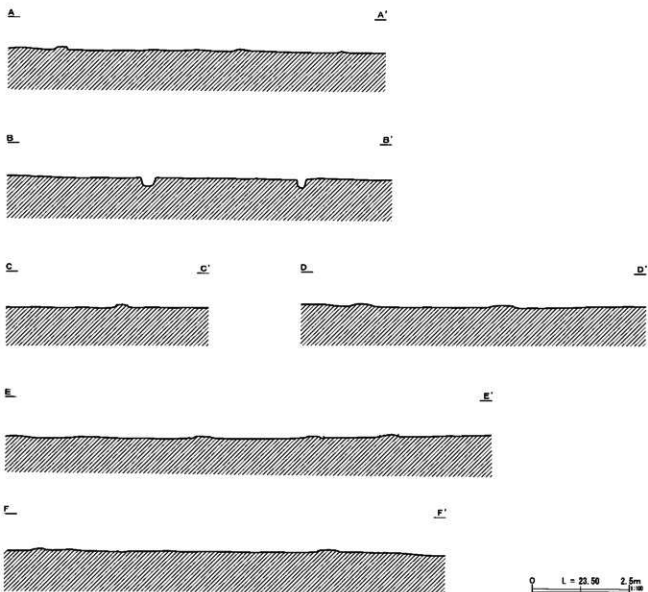
第179図 A区二面水田跡エレベーション図
