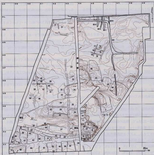
第189図 A区一面水田跡等高線図
