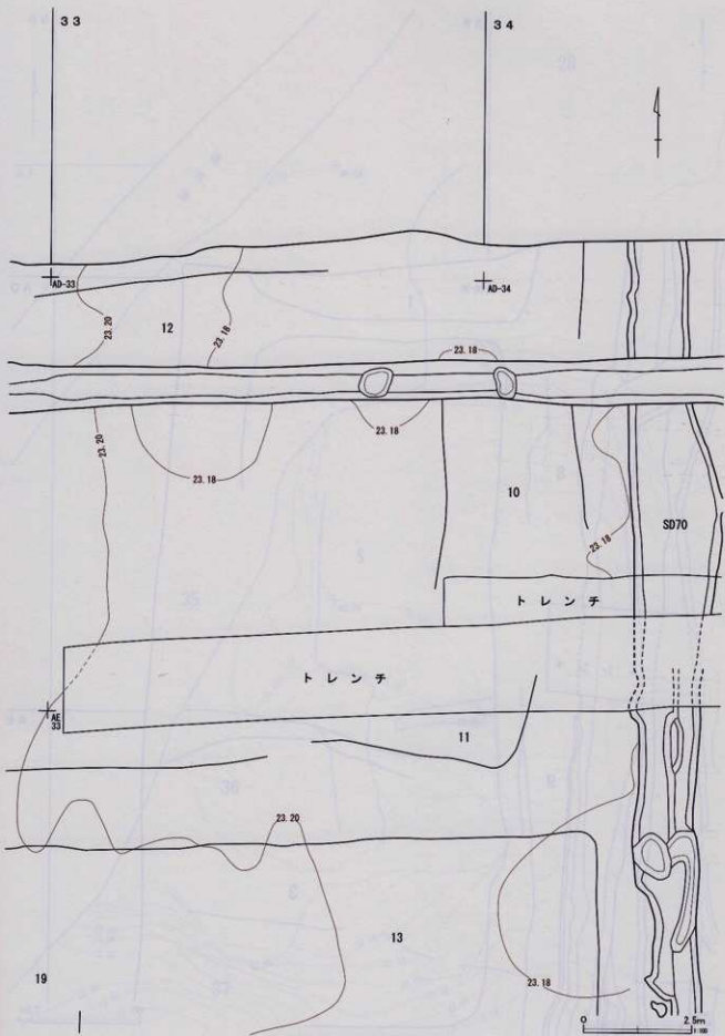
第243図 C区水田跡 (4)
