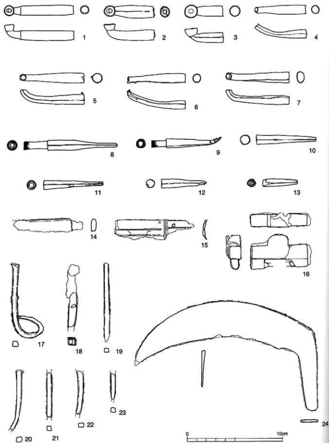
第62圖 金屬製品 (S=1/2)
