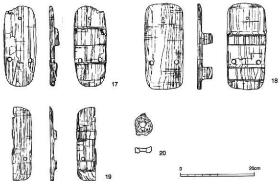
第64図 木製品(2) (S=1/5)
