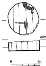
第7図 1号埋桶 (S=1/40)
