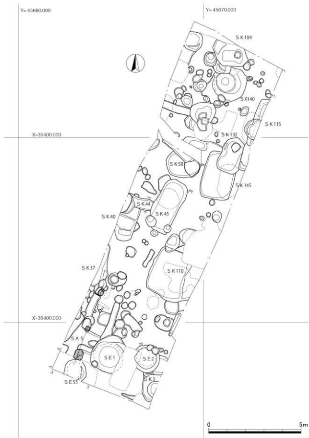
第3圖 遺構配置図 (1/100)
