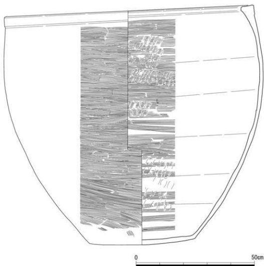
第9図 S X 140実測図 (1/40)
