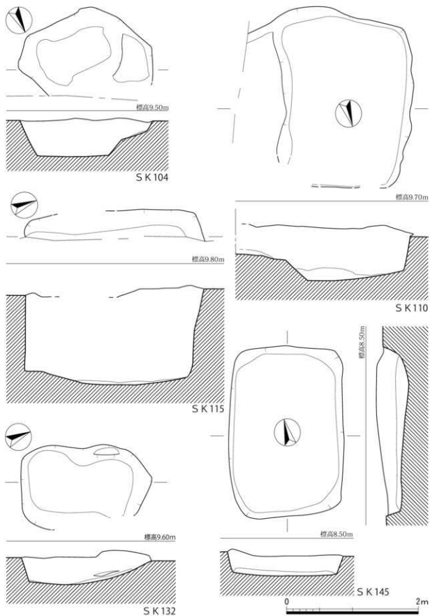
第7図 SK104・110・115・132・145実測図 (1/40)
