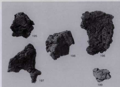
第3号炉出土炉壁・羽口・鉄滓(1) 第34図
