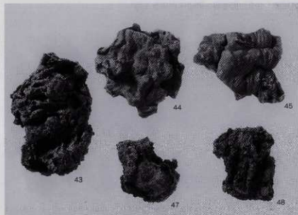
第1号炉出土炉壁·鉄滓類(6) 第18・19图
