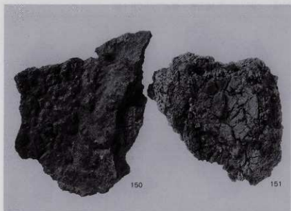
第2号炉出土炉壁·羽口(1)
