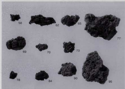
第1号炉出土炉壁·鉄滓類(7) 第19・20图
