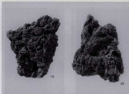
第1号炉出土炉壁·鉄滓類(3) 第16図
