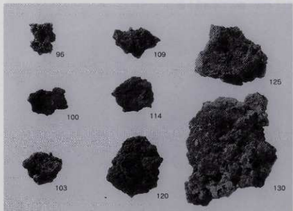
第1号炉出土炉壁·鉄滓類(8) 第20・21图
