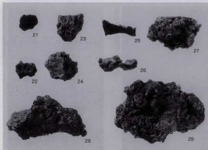
第1号炉出土炉壁·鉄滓類(4) 第16図
