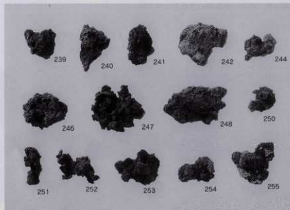
第3号炉出土炉壁・羽口・鉄滓(2)
