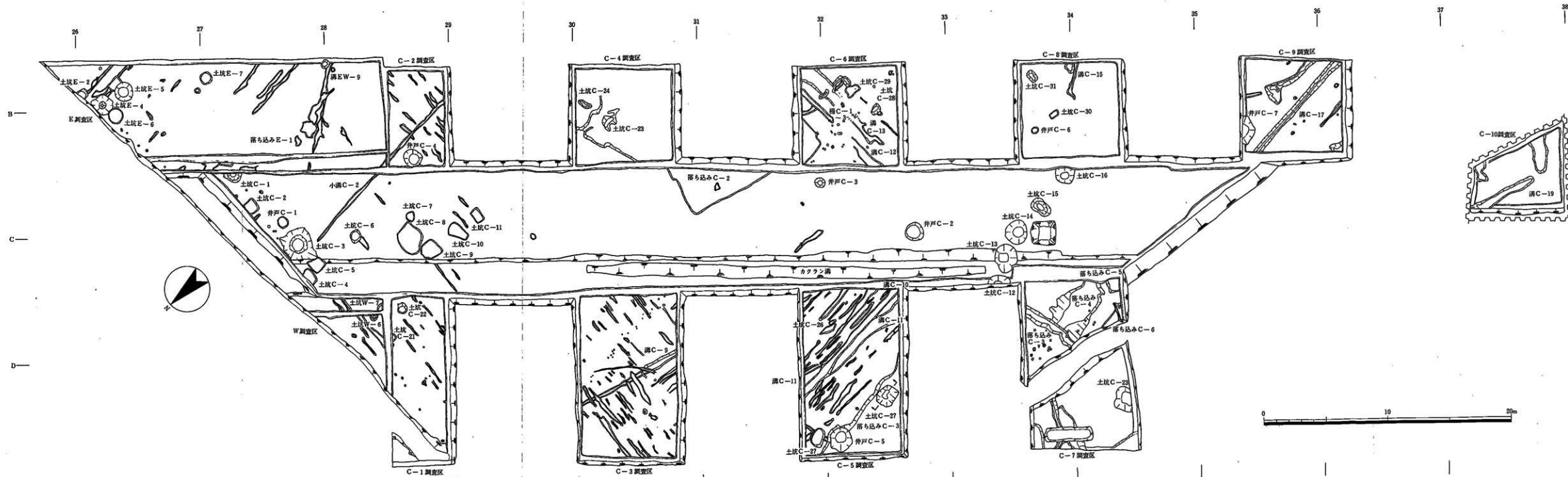
付図五 C調査区第1遺構面全体図 (1/200)
