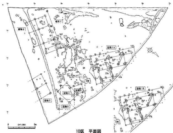
10区 平面図
