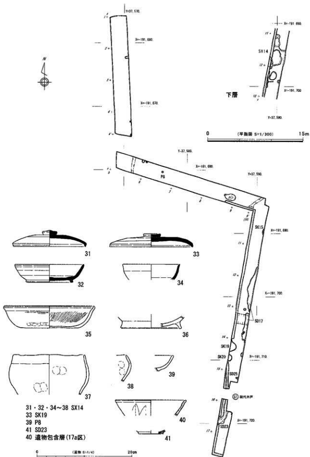
3区 平面図・出土遺物
