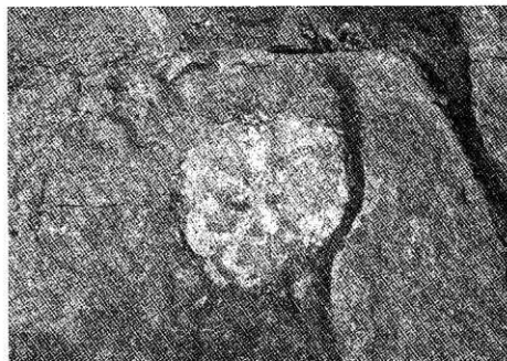
3. 化石産出状況 (ウニ類)
