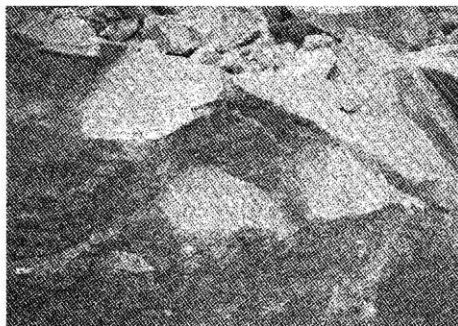
3. 化石産出状況 （アシヤニシキ）
