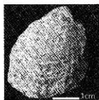
31. Venericardia subnipponica Nagao
