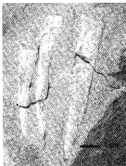
9. Dentalium ashियाensis (Nagao) 掘削岩塊 OTA-05080203
