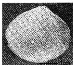
36. Macoma optiva (Yokoyama) 掘削岩塊 OTA-05082513
