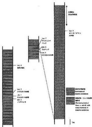
第4図 調査地域における化石産出層準
