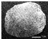
41. Pitar ashhyaensis (Nagao) 掘削岩塊 OTA-05082515
