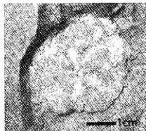
45. Linthia praenipponica Nagao B区面 Loc. 6 OTA-05082519
