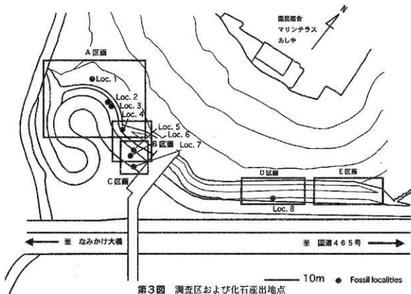
第3図 調査区および化石産出地点
