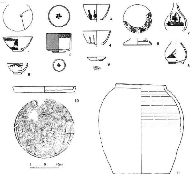
図16 B区1号土坑出土遺物 (S-1/4)
