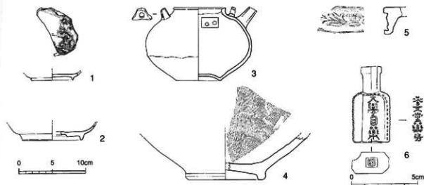
図4 A区出土遺物(1~5はS=1/4、6はS=1/2)
