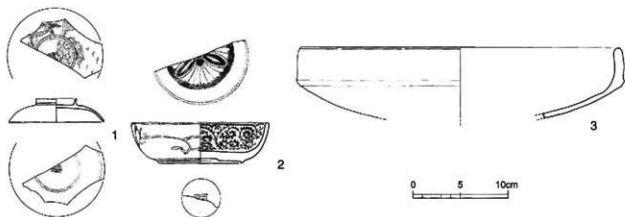
図11 トレンチ内6層出土遺物 (S=1/4)
