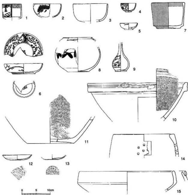
図10 B区6層遺物集中部出土遺物 (S=1/4)
