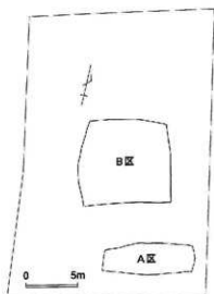
図2 調査区位置図 (S=1/400)
