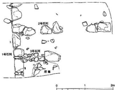
図3 A区遺構配置図 (S=1/40)
