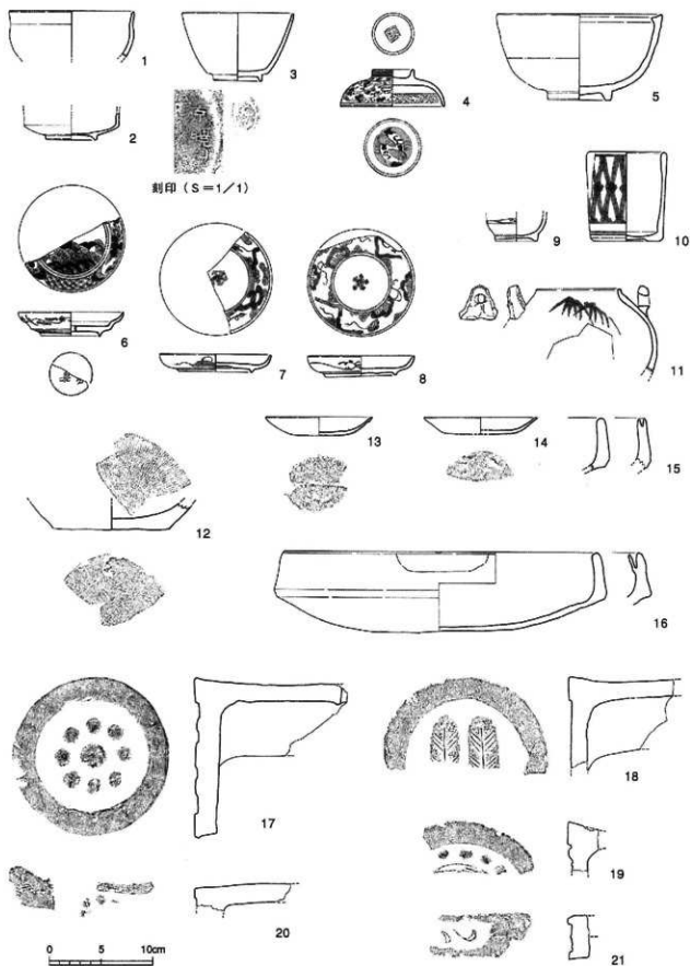
图15 B区1号瓦溜出土物 (S=1/4)
