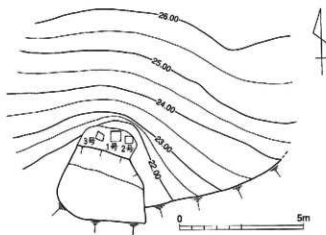
第9図 萩山石塔配置図(S=1/150)
