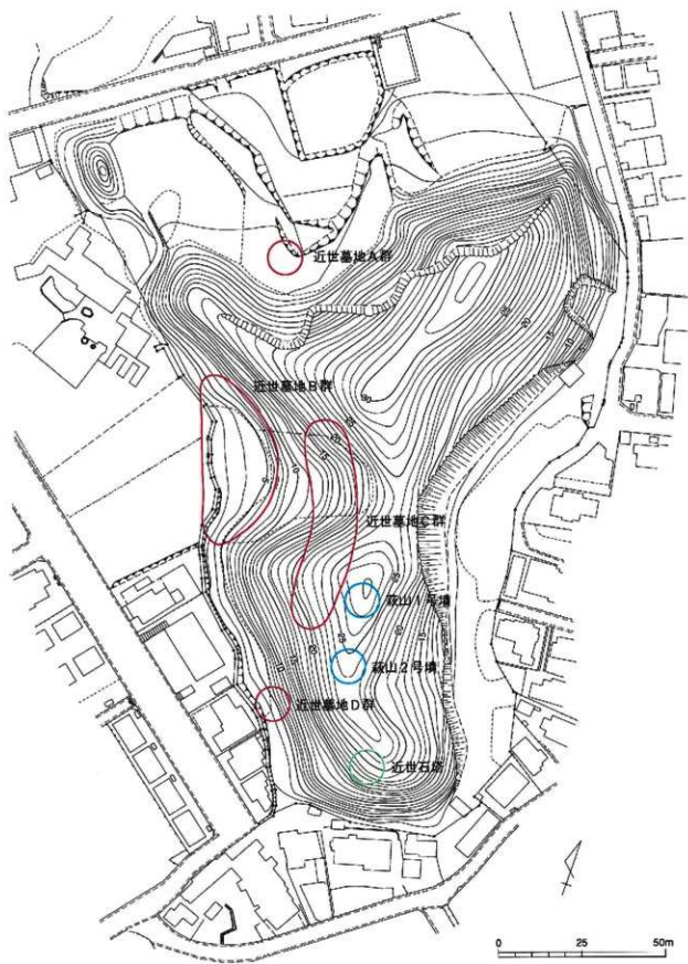
第2図 萩山遺跡群周辺地形図 (S=1/1250)
