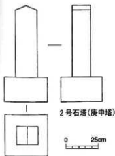
第10図 萩山石塔実測図(S=1/20)
