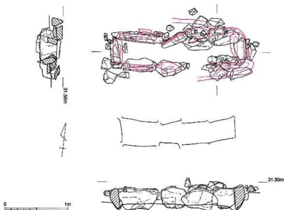
第4図 1号墳主体部実測図（S=1/30）
