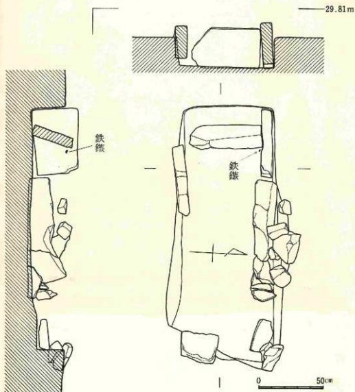
6図 2号棺実測図
