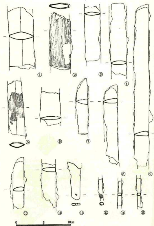
8图 铁剑、铁刀、铁镞实测图
