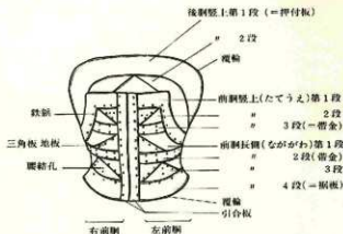
10図 短甲各部の名称
