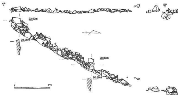
第5図 1号石垣実測図 (S=1/60)
