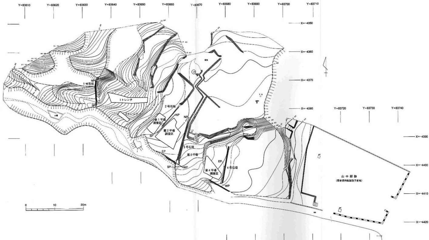
第6図 山中家屋敷跡・竹中家屋敷跡周辺地形測量図と調査区位置図 (S=1/400)
