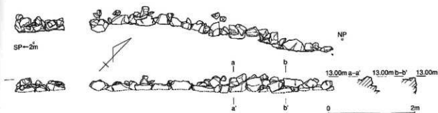
第7図 2号石垣実測図 (S=1/60)
