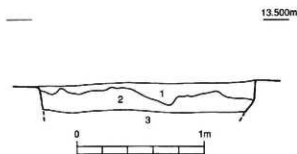
第3図 第2平場北東壁土層図 (S=1/30) 1層: 黒色土(腐葉土)…表土 2層: 茶褐色土、ハード…近世の整地層 第1平場3層と同一 3層: 明茶褐色土(レキ混層)
