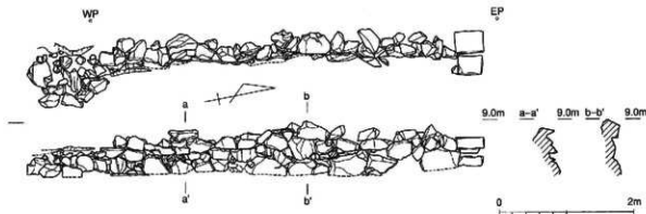
第8図 4号石垣実測図 (S=1/60)
