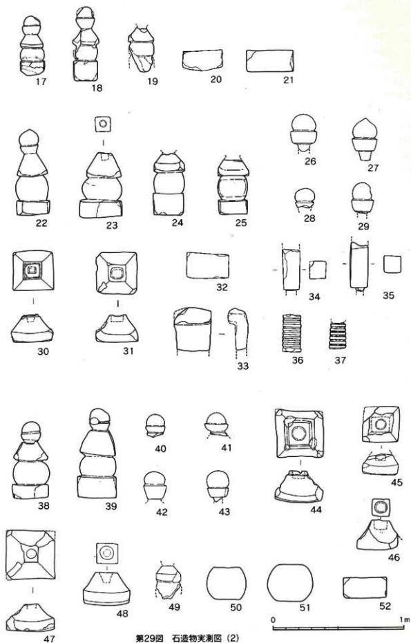
第29图 石造物実測图 (2)
