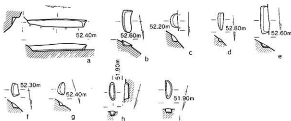
第13図 掘り込み実測図
