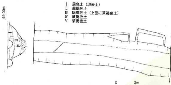
第4図 溝実測図
