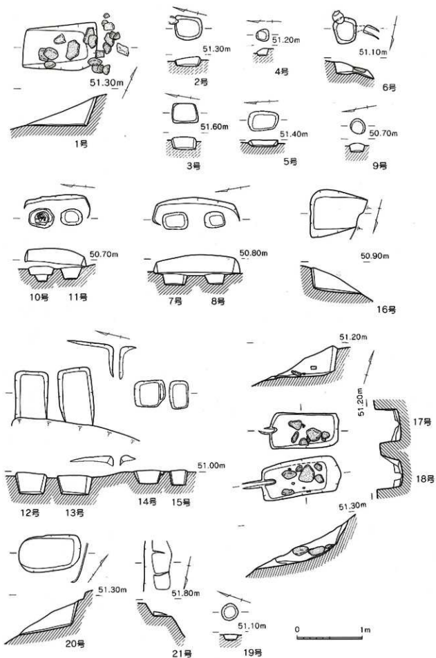
第10图 墓坑实测图(1)
