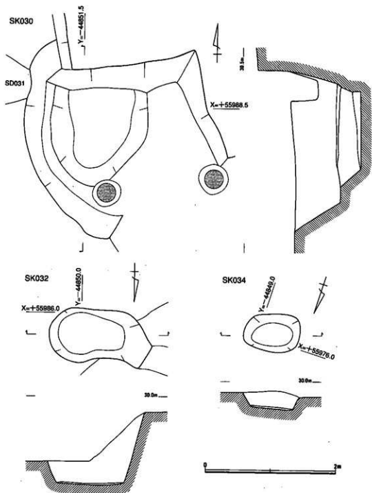
第14图 212SK030·032·034实测图(1/40)
