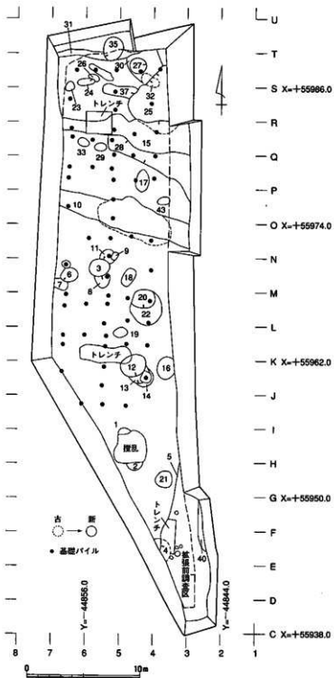
第33図 212次調査略測図 (1/300)
