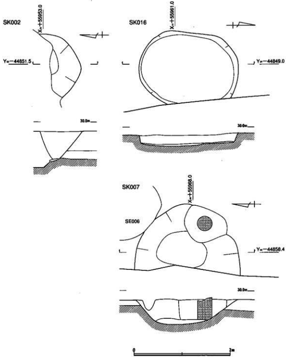
第11图 212SK002·007·016实测图(1/40)
