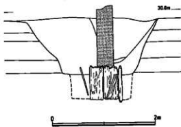
第10图 212SE022实测图 (1/50)
