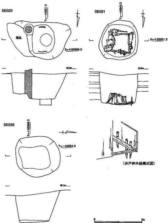
第9図 212SE020・021・035実測図(1/50)
