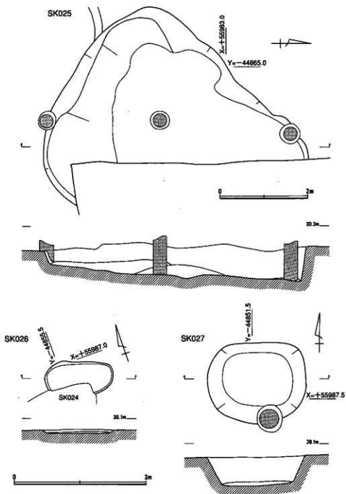
第13图 212SK025~027实测图 (1/40 · 1/60)
