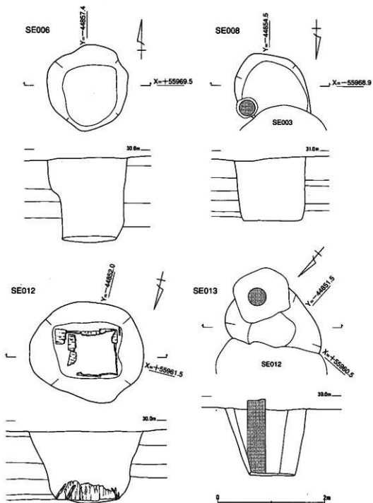
第 8 图 212SE006 · 008 · 012 · 013 实测图 (1/50)
