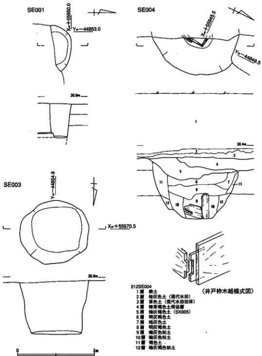
第7圖 212SE001・003・004実測圖 (1/50)
