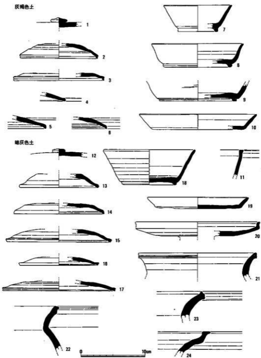
第29图 212SK030出土遺物実測图1 (1/3)
