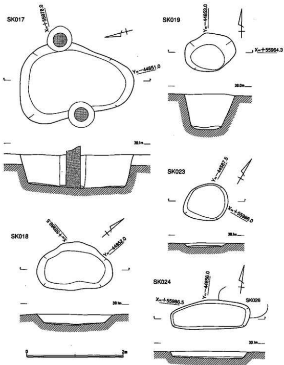
第12図 212SK017~019・023・024実測図(1/40)
