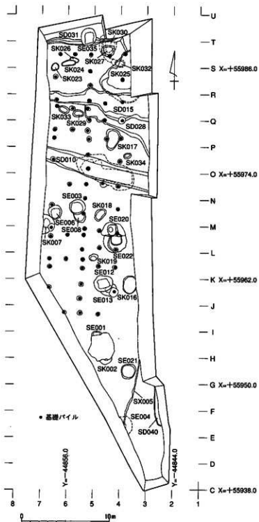
第3図 212次調査遺構配置図 (1/300)
