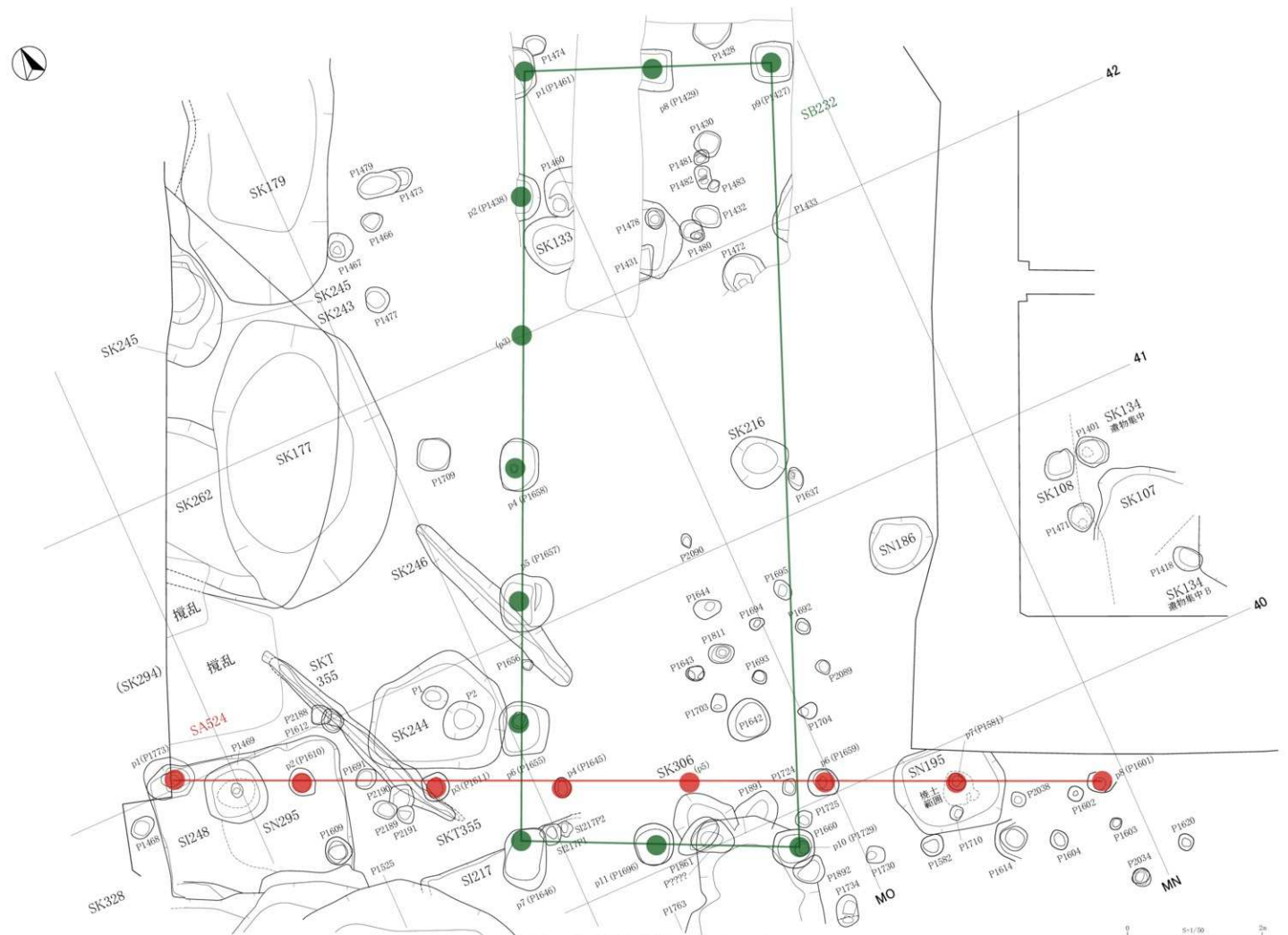
付图 8 掘立柱建物跡④ (S B 232 S A 524)
