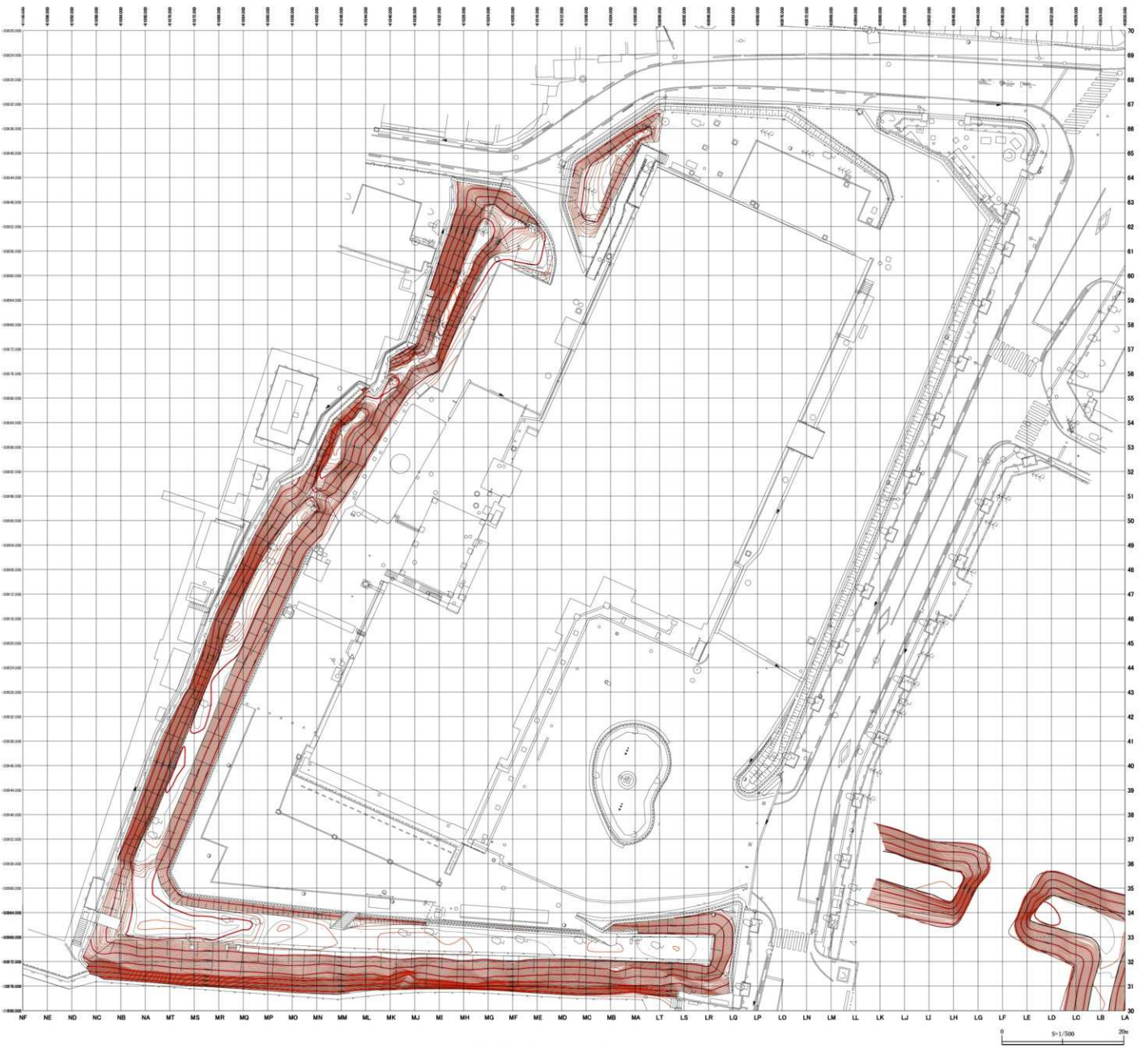
付図14 久保田城跡 土塁測量図
