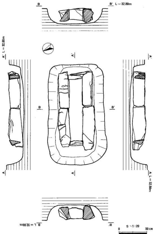
插图 8 箭溪18号墳第2号埋葬施設(石棺)実測図
