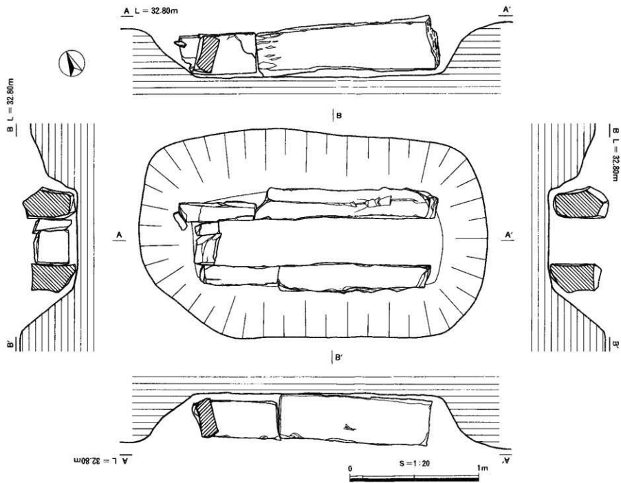
挿圖7 箭浜18号墳第1号埋葬施設(石棺)実測図
