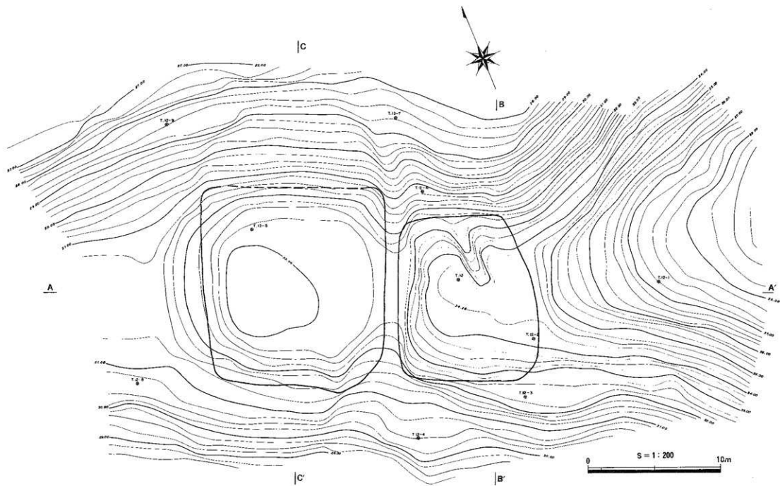
插图 4 箭溪 18·19 号填地形实测图
