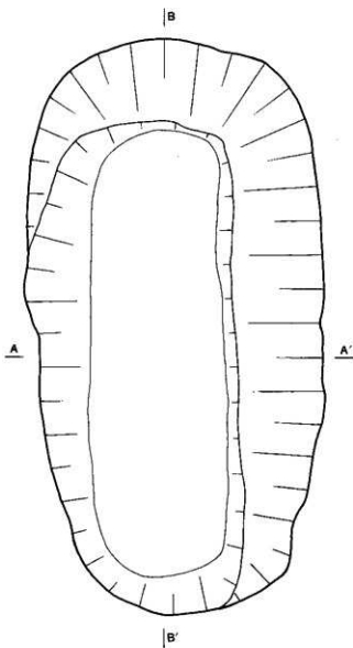
挿圖14 箭溪19号墳埋葬施設(木棺)実測図
