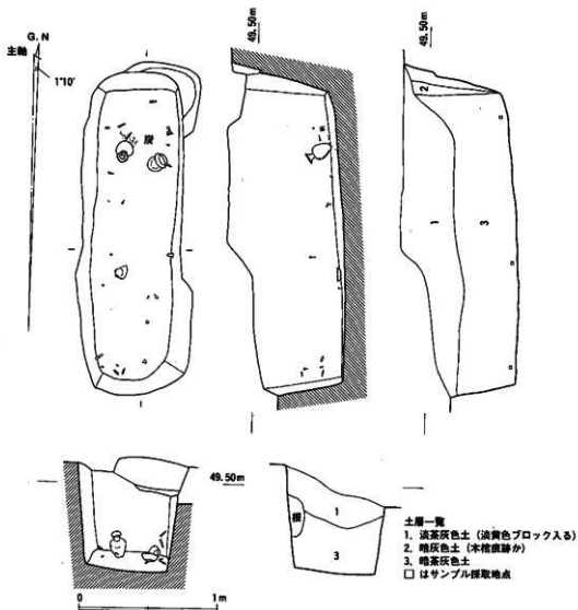
Fig. 42 7ST002 実測図 (1/30)
