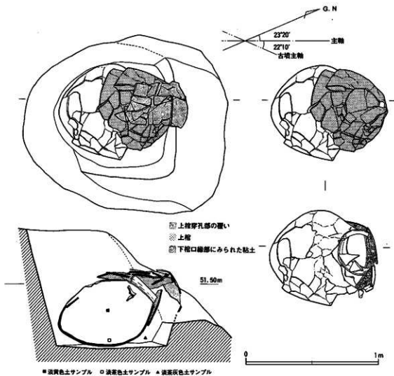
Fig. 28 7ST100 実測図 (1/20)
