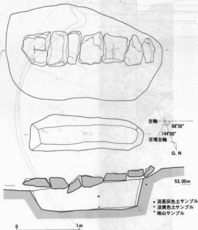
Fig. 34 7ST020 実測図 (1/30)
