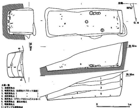
Fig. 49 7ST030 実測図 (1/30)
