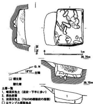
Fig. 62 7SX045 実測図 (1/30)
