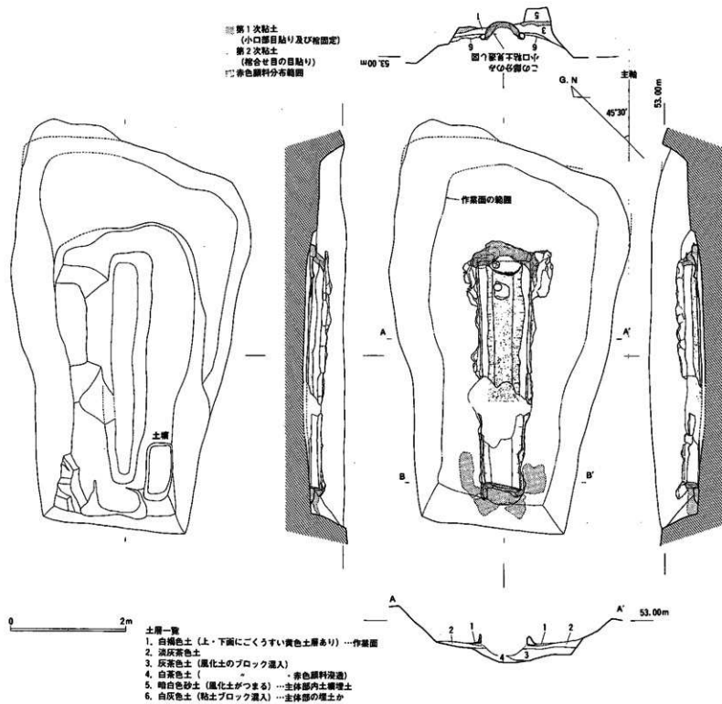
Fig. 8 12号墳主体部実測図 (1/60)
