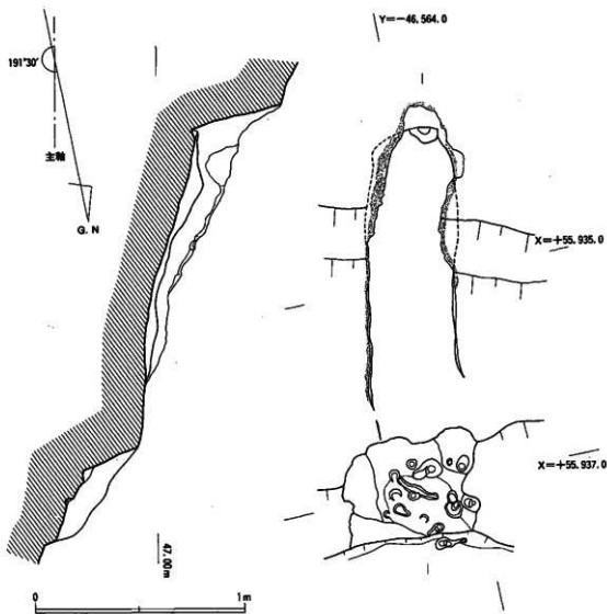
Fig. 37 10号窟実測図 (1/40)
