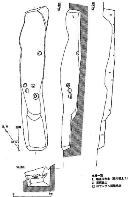
Fig. 43 7ST003 実測図 (1/30)
