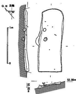
Fig. 46 7ST015 実測図 (1/30)
