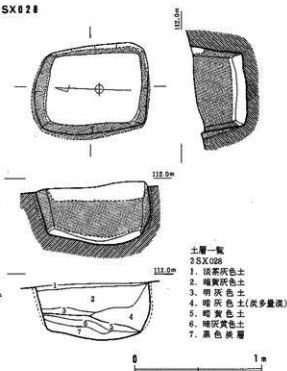
Fig. 21 K区検出焼土墳実測図(III)
