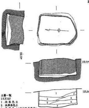
Fig. 21 K区検出焼土墳実測図(III)
