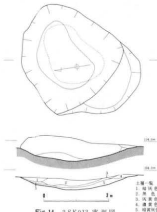
Fig. 14 2SK013 実測図
