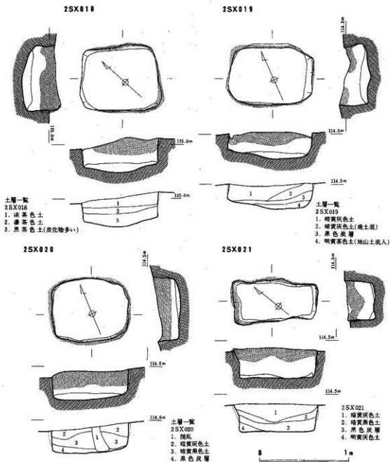
Fig. 19 K区検出焼土坑実測図 (I)
