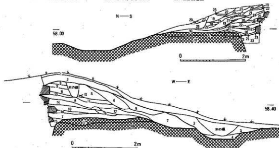
Fig 3. 墳丘土層図 (1/60)
