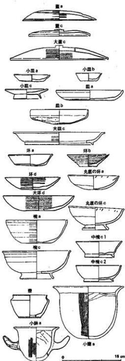
図17-1 土師器の器種分類 (1/5)
