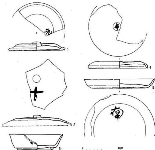
図22 第6トレンチ出土墨書土器 (1/3)
