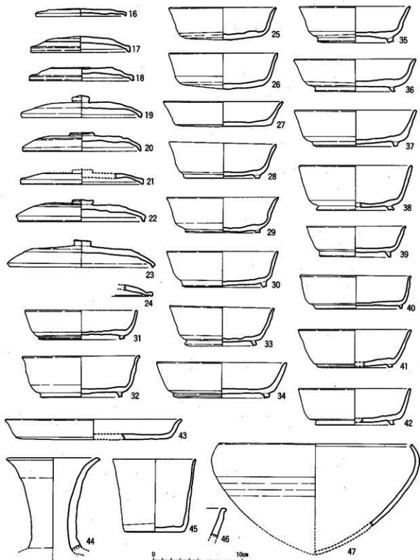
圖21 SD001下層出土土器 (1/3)
