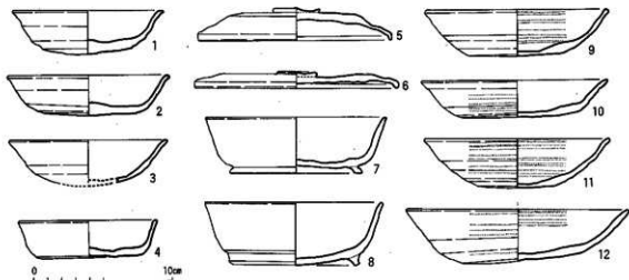
図19 包含層出土土器 (1/3)
