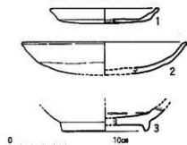
図25 SE005出土土器 (1/3)
