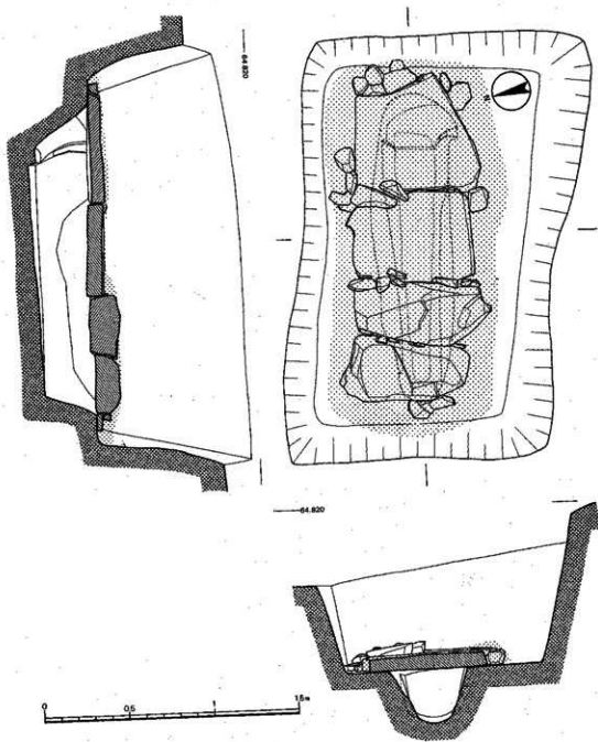
第20图 6号主体部通槨实测图
