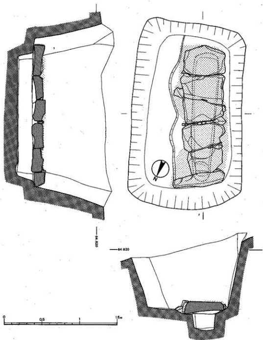
第23图 7号主体部遺構実測図
