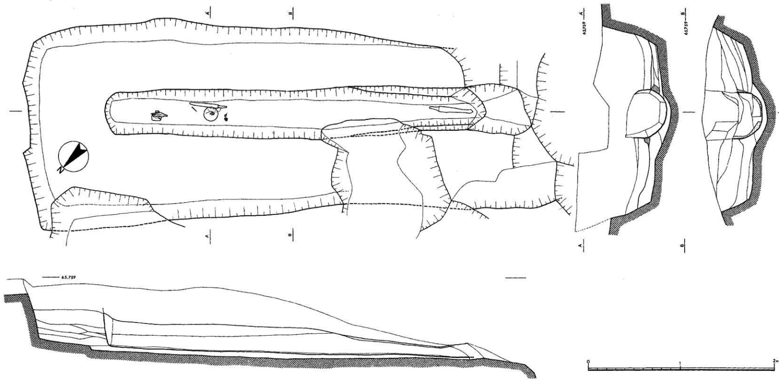
第8图 1号主体部实测图
