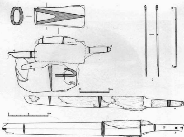
第13图 铁斧，刀子，箭，铜先，铁刀，铁刺尖测图
