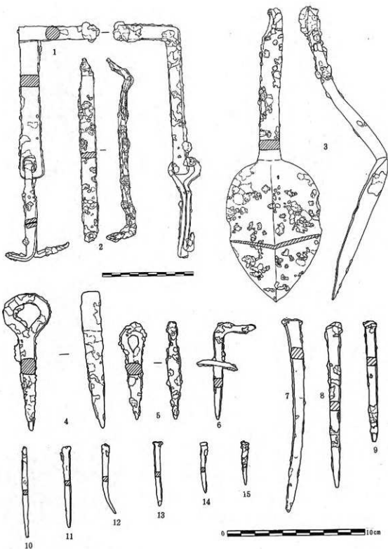
第11图 铁製品・角釘実測図
