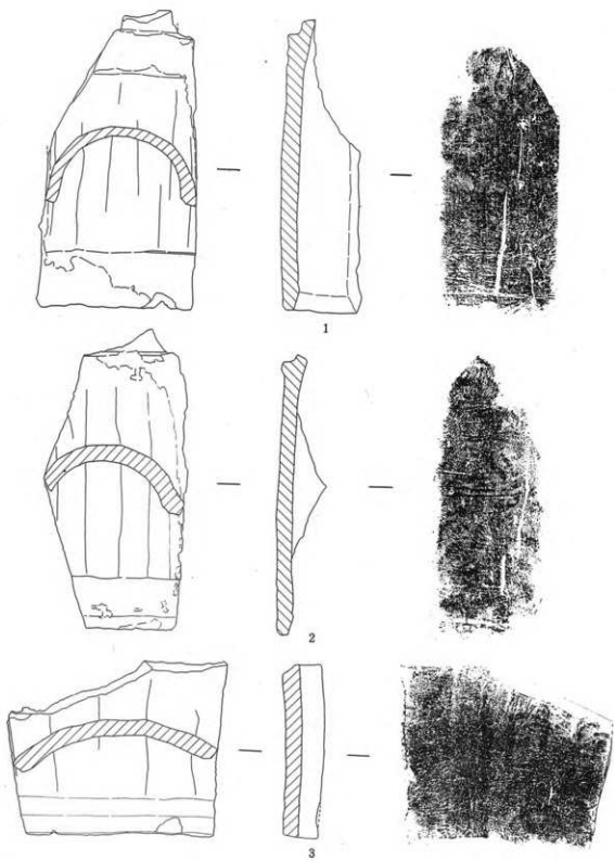
第10图 丸瓦・平瓦实测、拓影
