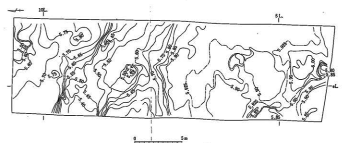
付図1 調査区割付図 (上) Aトレンチ弥生時代中期遺構面平面図 500 (下左) Aトレンチ弥生時代後期遺構面平面図 500 (下中) AトレンチN R 6001河床面平面図 500 (等高線間隔5cm 下右)
