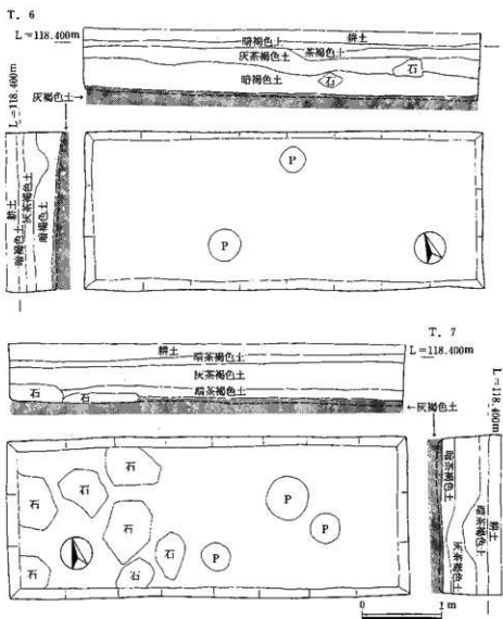
第6図 トレンチ平面・断面図
