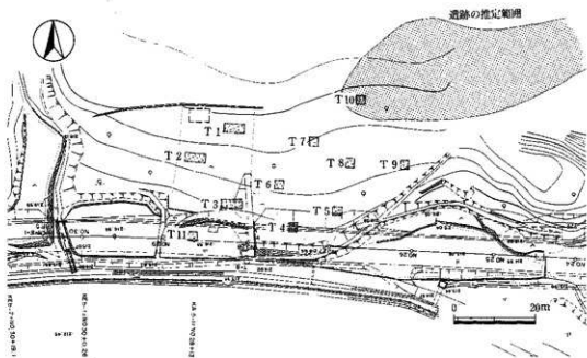
第15図 イヤノ谷遺跡トレンチ配置図
