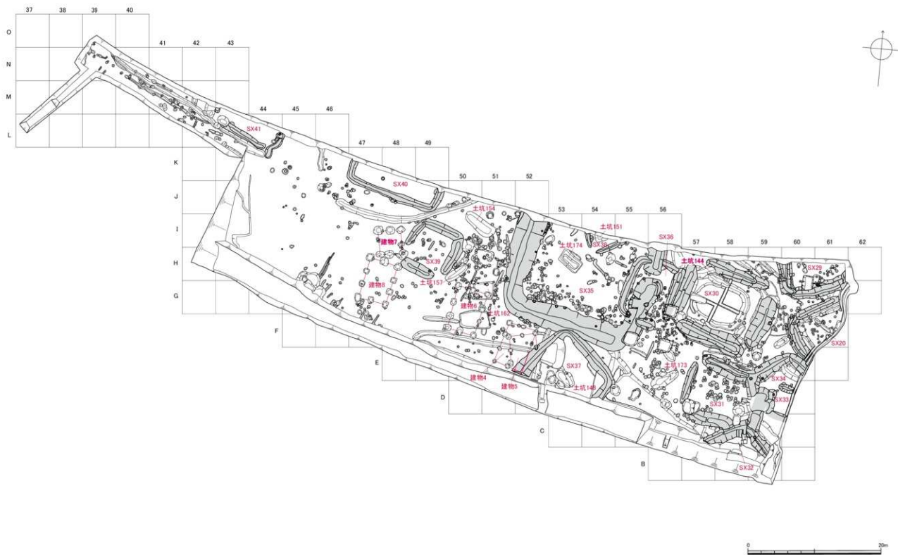
第11圖 調査Ⅱ区下層遺構図 (3) 平成15・16年度 (縮尺1/400)
