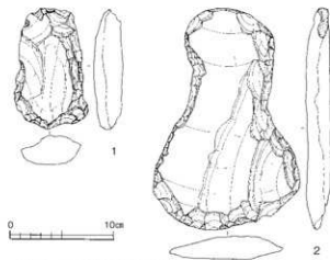
第10図 石器実測図 (縮尺1/4)
