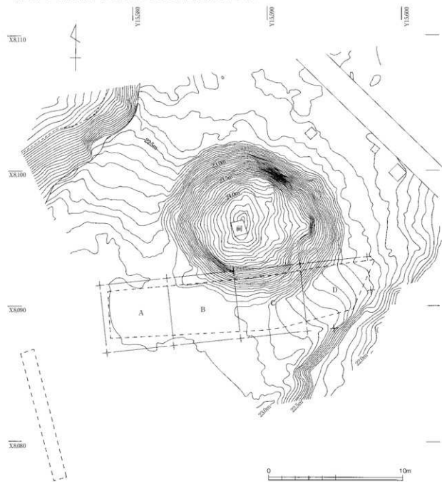
第2図 調査区およびグリッド配置図（縮尺1/200）
