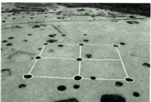
F 区第75号掘立柱建物跡
