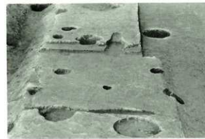
F区第120号住居跡
