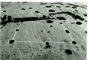
F 区第54号掘立柱建物跡
