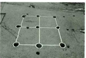
F 区第62号掘立柱建物跡
