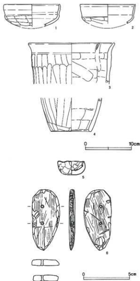
第523図 G区第5号住居跡出土遺物
