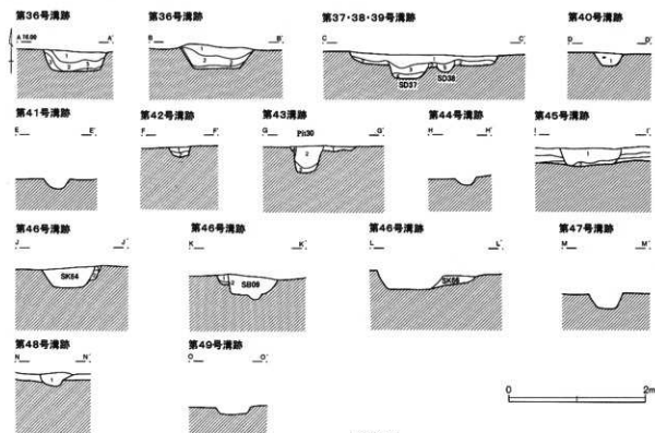
第571図 G区溝跡(6) (第517図)
