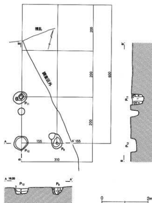
第543図 G区第8号掘立柱建物跡
