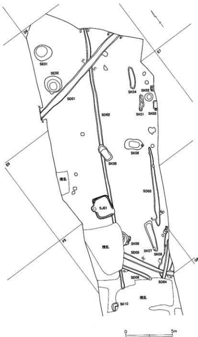
第512図 G区全体図(1)
