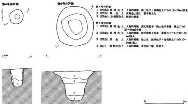
第562图 G区井戸跡(3) (第515回)
