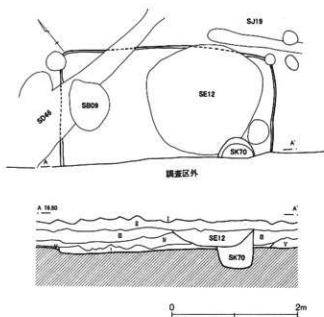
第535図 G区第21号住居跡
