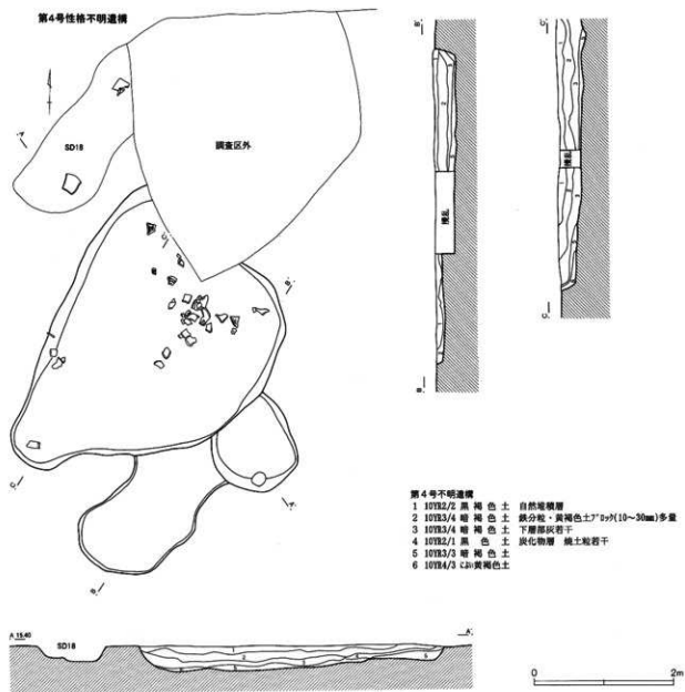
第575図 G区性格不明遺構(2)
