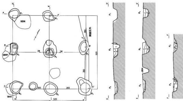
第540図 G区第5号掘立柱建物跡
