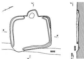
第518図 G区第1号住居跡
