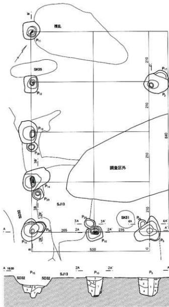
第541図 G区第6号掘立柱建物跡
