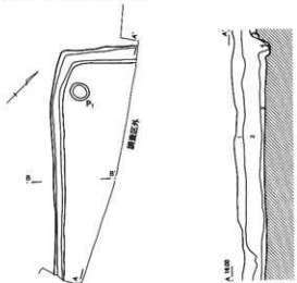
第519図 G区第3号住居跡
