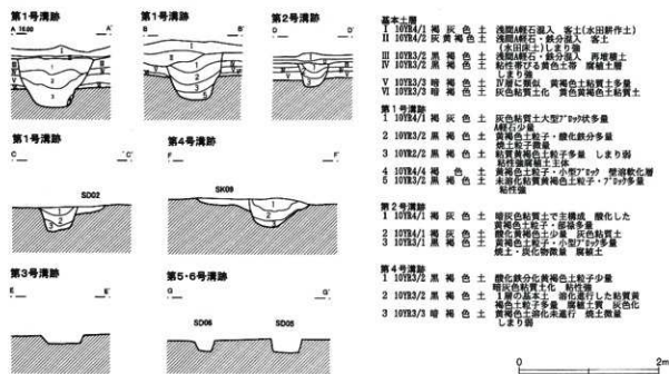
第566図 G区溝跡(1) (第512図)
