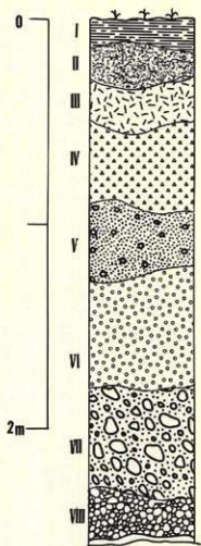
第5図 基本層序柱状図
