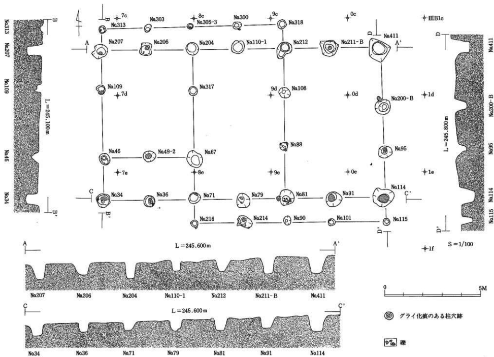
第10図 第1号直立柱建物跡
