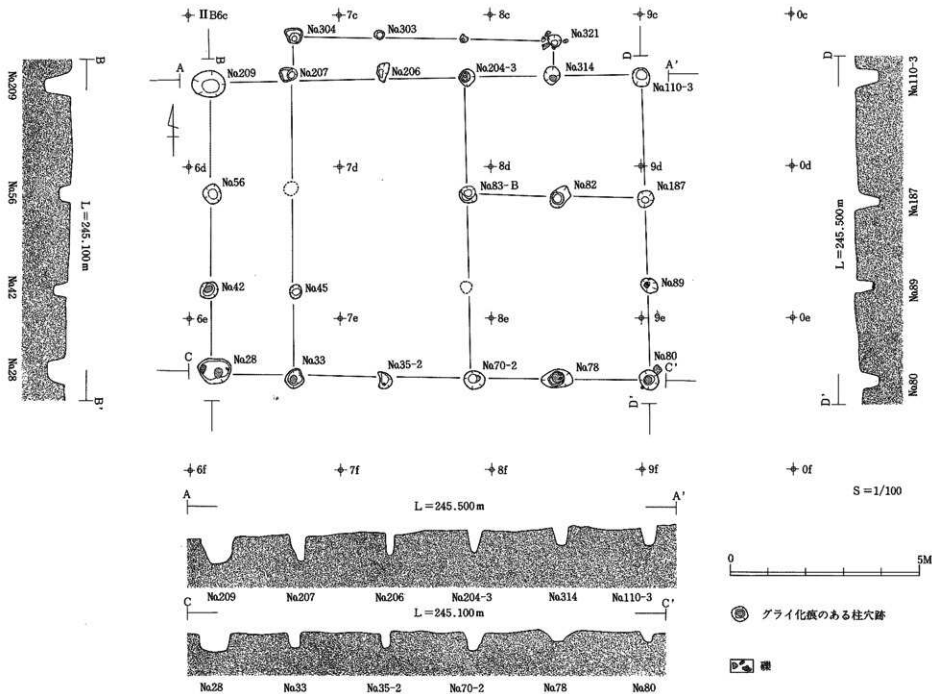
第11図 第2号竪立柱建物跡
