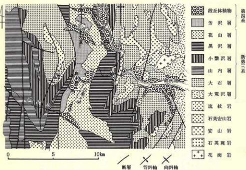
第4図 平鹿盆地付近の地質図 (長谷地質調査事務所(1981)による)
