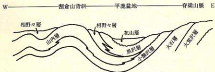
第3図 平鹿盆地の東西両縁部を含む東西断面図 (長谷地質調査事務所(1983))
