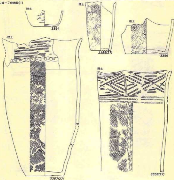
第173图 JⅦ-6·JⅦ-7住居址
