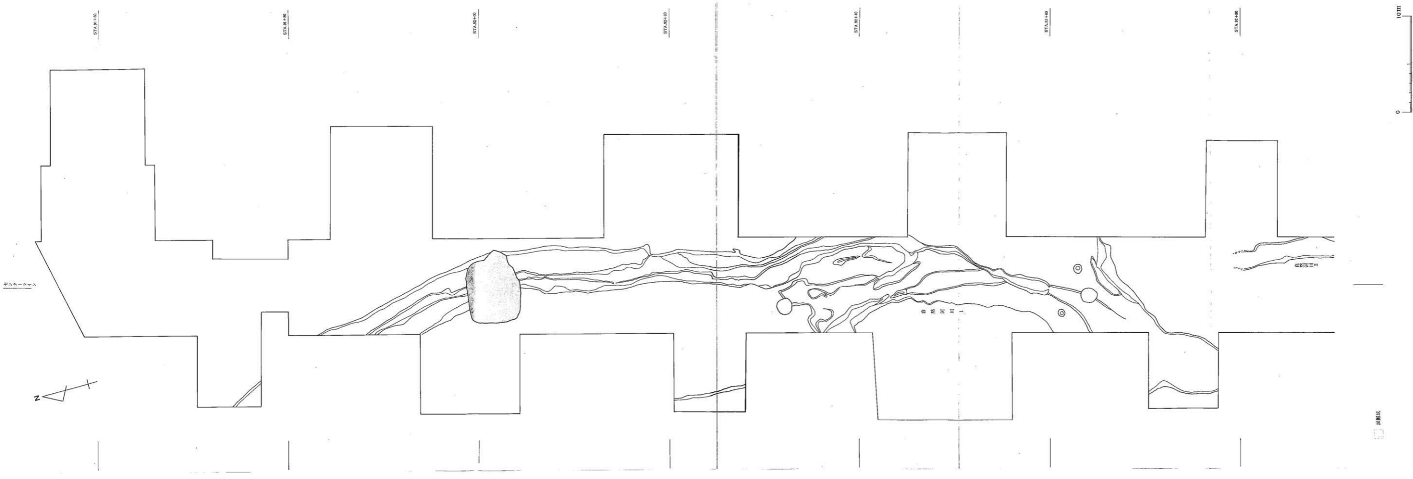
付図15 古墳時代後期全体図① (1/500)
